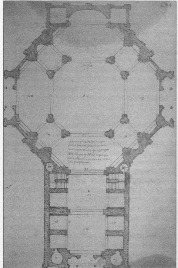
Fig. 10. Hernán Ruiz II. Proyecto de templo. Folio 104 del Libro de arquitectura.
