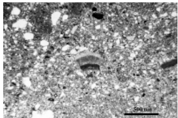
Figura 3. Fotografía al microscopio óptico de restos fósiles detectados en la muestra L8
