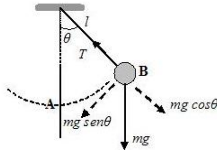
Figura 2 Péndulo simple
