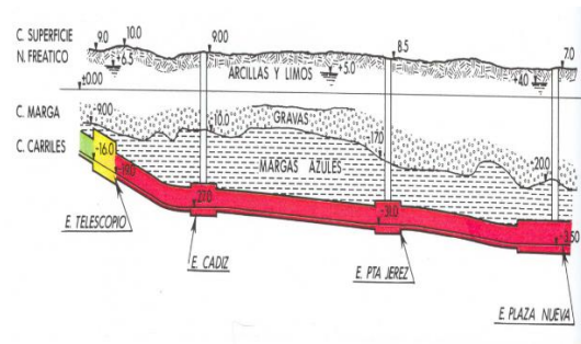
Figura 4. Telescopio – Plaza Nueva
