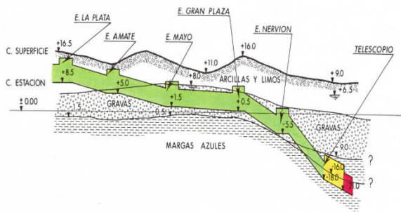
Figura 3. La Plata – Telescopio
