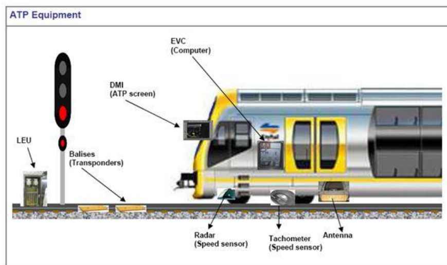
Figura 16. Resumen del equipamiento del ATP.
