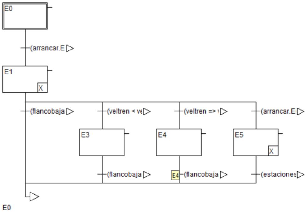
Figura 24. Secuencia del programa dinámica.
