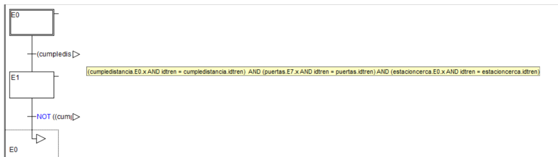
Figura 23. Secuencia del programa arrancar.
