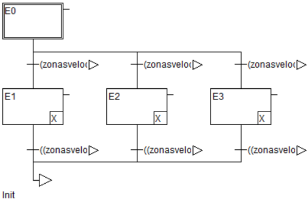
Figura 25. Secuencia del programa zonasvelocidad.
