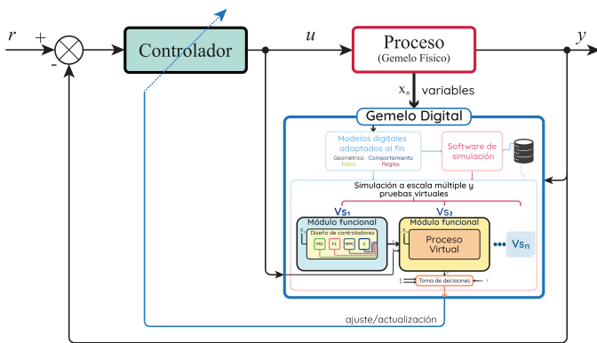
Figura 4: Gemelo digital usado para diseño de controlador
