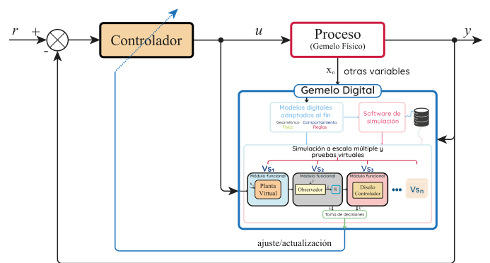
Figura 6: Observador dentro de un Gemelo Digital
