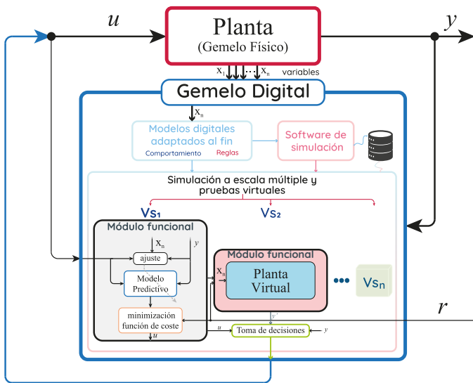
Figura 5: Esquema de MPC con actualización del modelo
