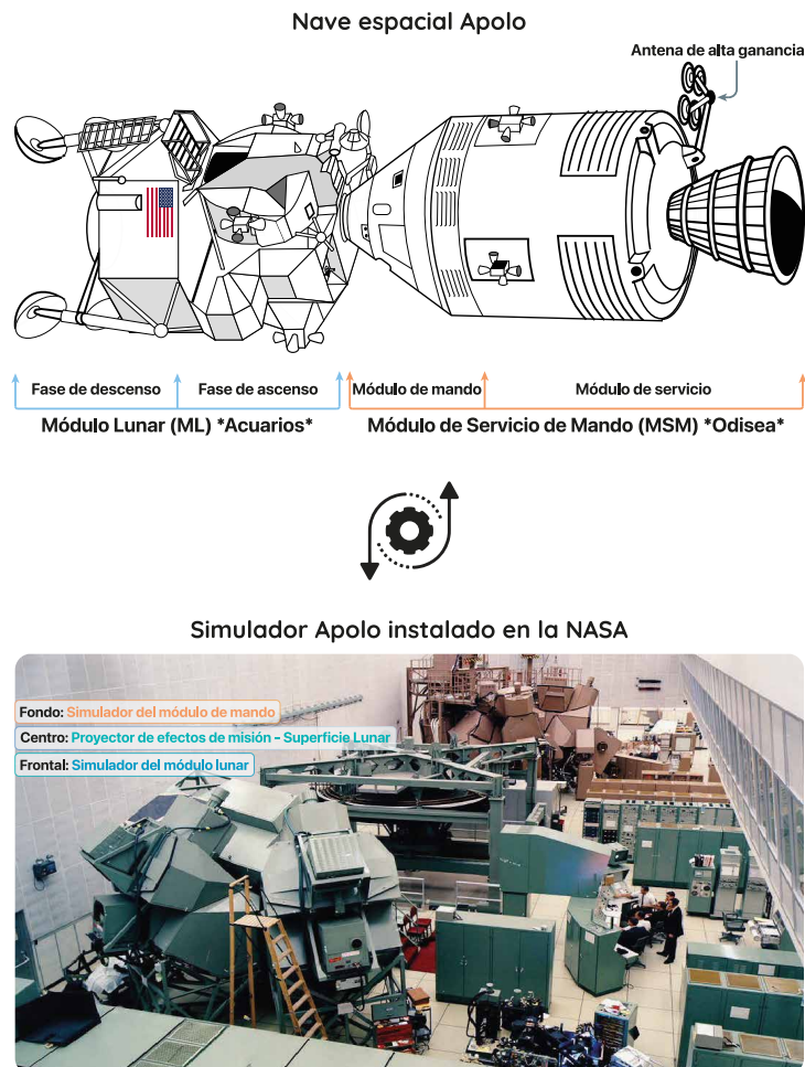
Figura 1: Primer modelo gemelo digital implementado en la Misión Apolo 13 de la NASA. Gráfico creado por el autor, con archivos de Wikimedia Commons de dominio público y una presentación de uso público de la NASA (Allen, 2021).
