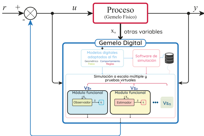
Figura 7: Actualización de observador mediante un Gemelo Digital
