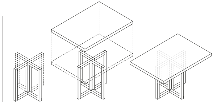
Axonometría mesa para 4
