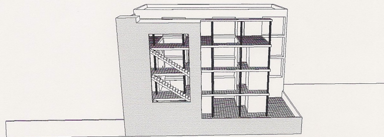
SECCION A-A'
