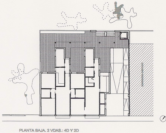
PLANTA BAJA. 2 VDAS.: 4D Y 2D
