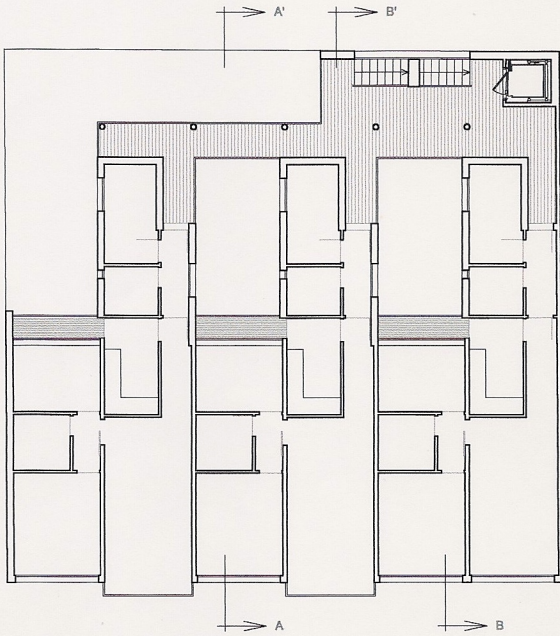
PLANTA 1ª Y 2ª. 3 VDAS.: 3D
