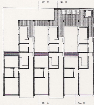
PLANTA 1ª Y 2ª. 3 VDAS.: 3D
