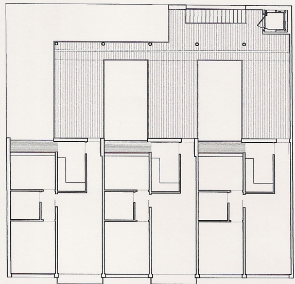
PLANTA 3ª. 3 VDAS.: 2D
