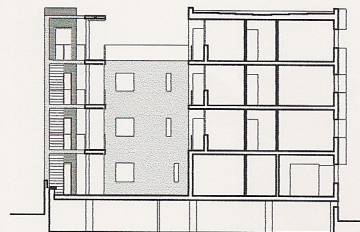
SECCION A-A'
