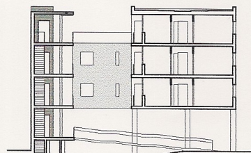
SECCION B-B'
