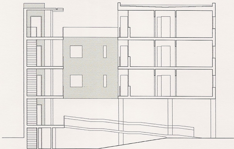
SECCION B-B'
