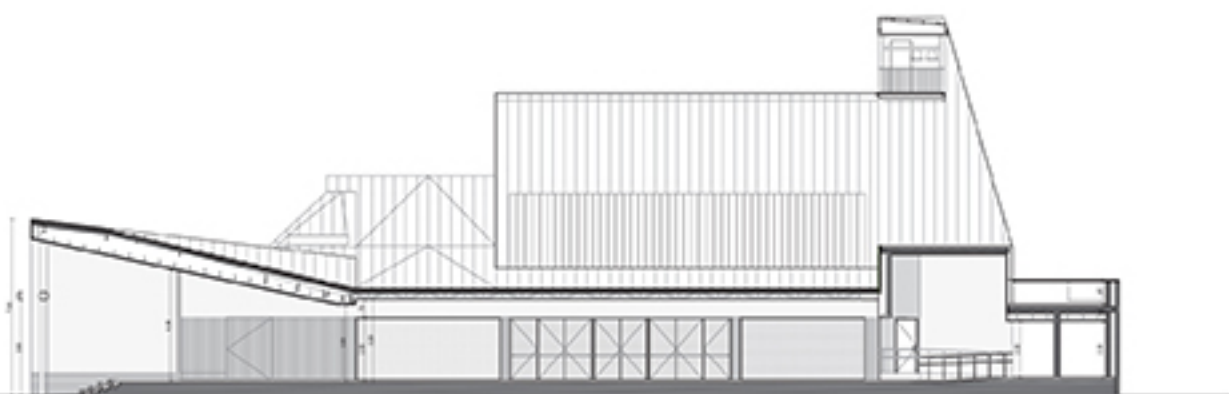
SECCIONES LONGITUDINALES
