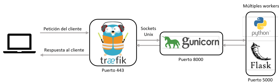
Figura 3.2 Esquema completo del sistema.
