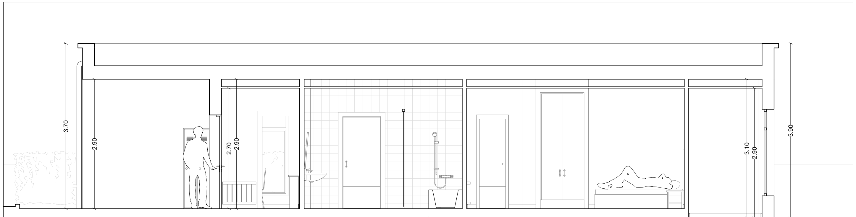
SECCIÓN LONGITUDINAL (1-1')
