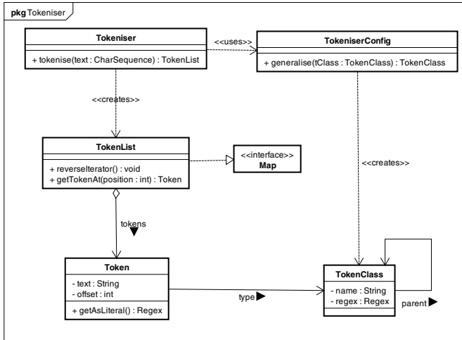
Fig. 2 Tokeniser
