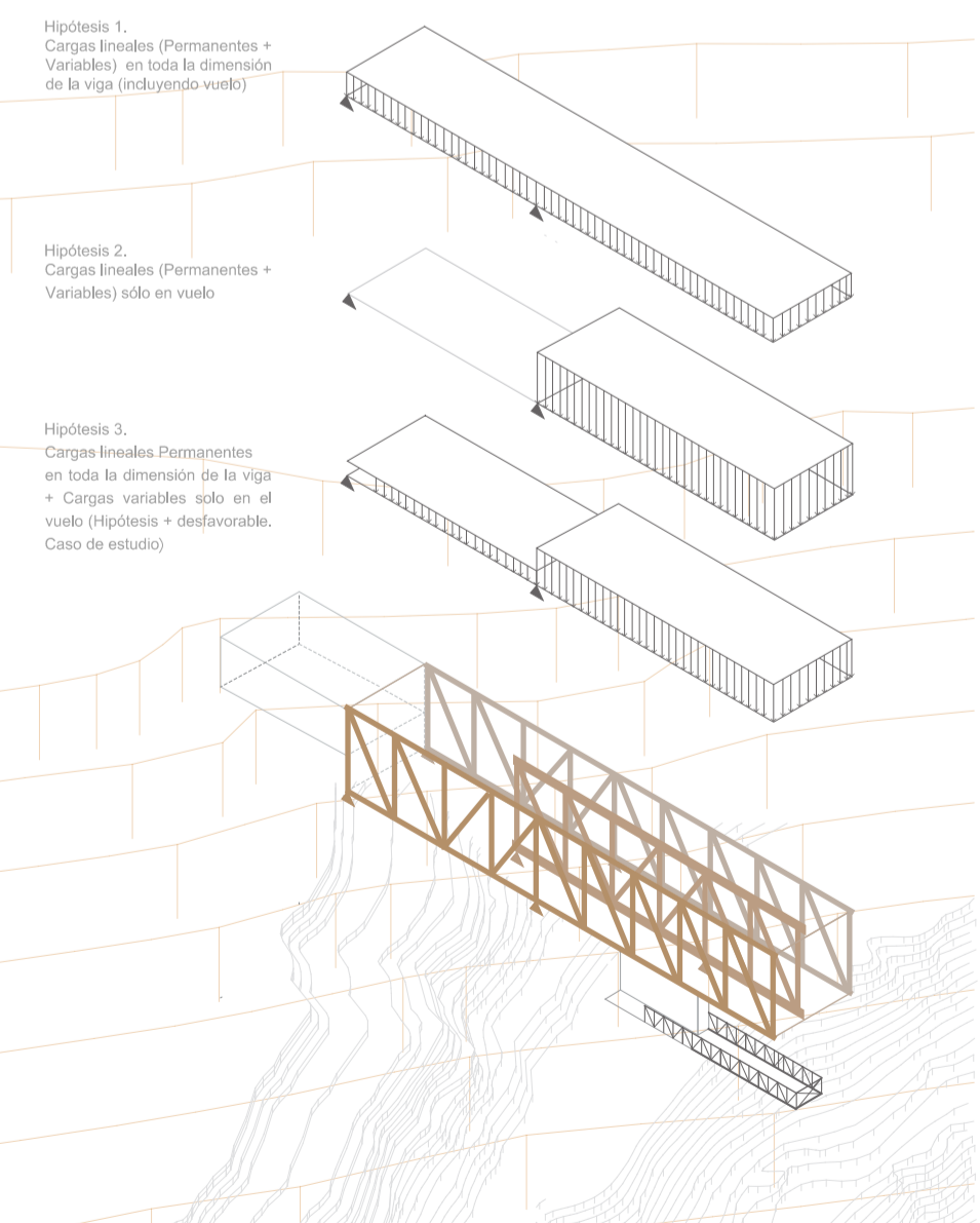
ESQUEMA DE ESTUDIO DE LA ESTRUCTURA METÁLICA Se hace necesario explicar una serie de consideraciones fundamentales que se han tenido en cuenta, con el objetivo de optimizar el cálculo y obtener unos resultados lo más ajustados y óptimos posibles. Se ha realizado un estudio intensivo acerca del funcionamiento de la estructura planteada, dependiendo la posición de la carga para el estudio del mismo. A continuación, se expone de forma esquemática el desarrollo que se ha seguido hasta elegir la hipótesis.
