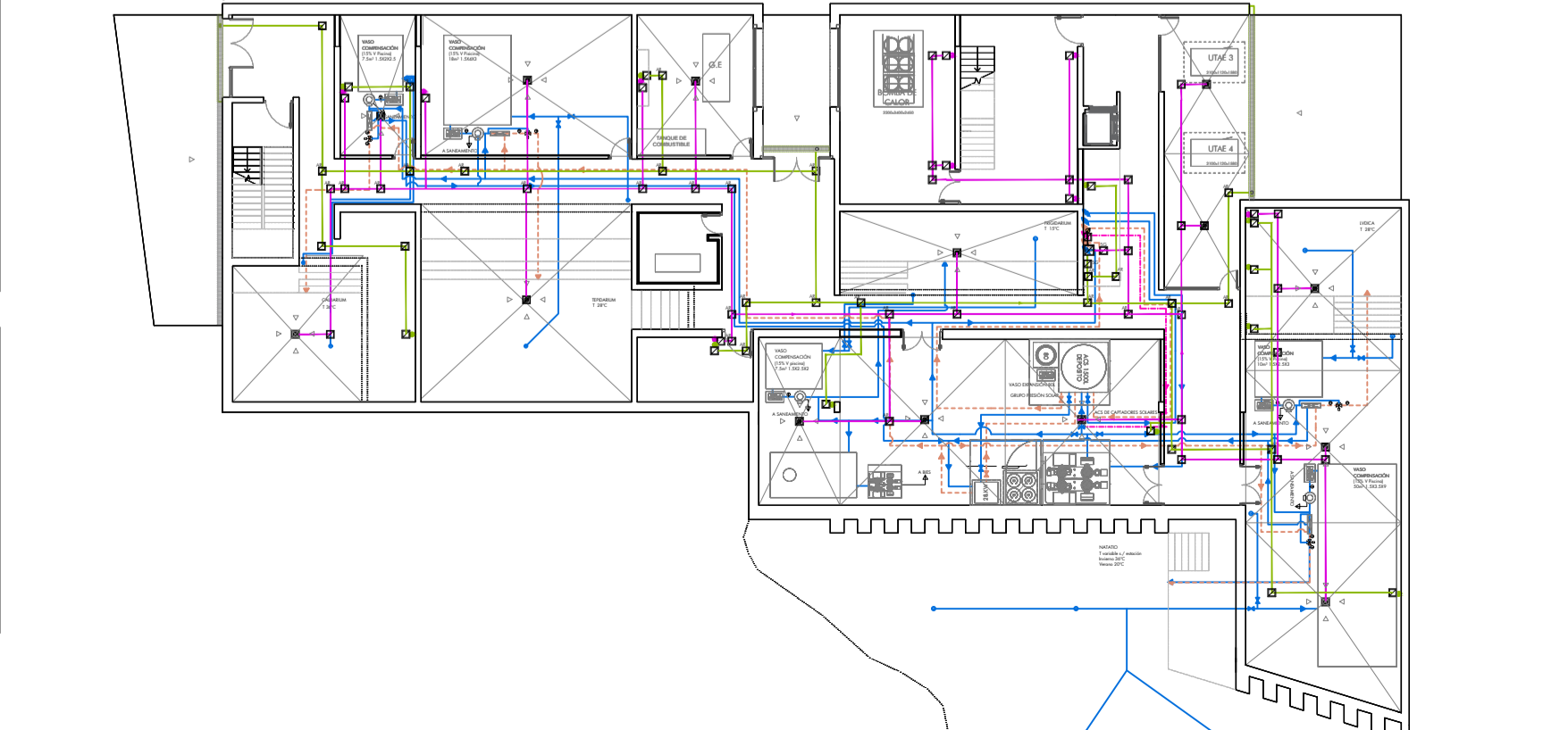
Instalación de ACS/AFS y saneamiento. Planta menos tres, nivel técnico... escala 1/300
