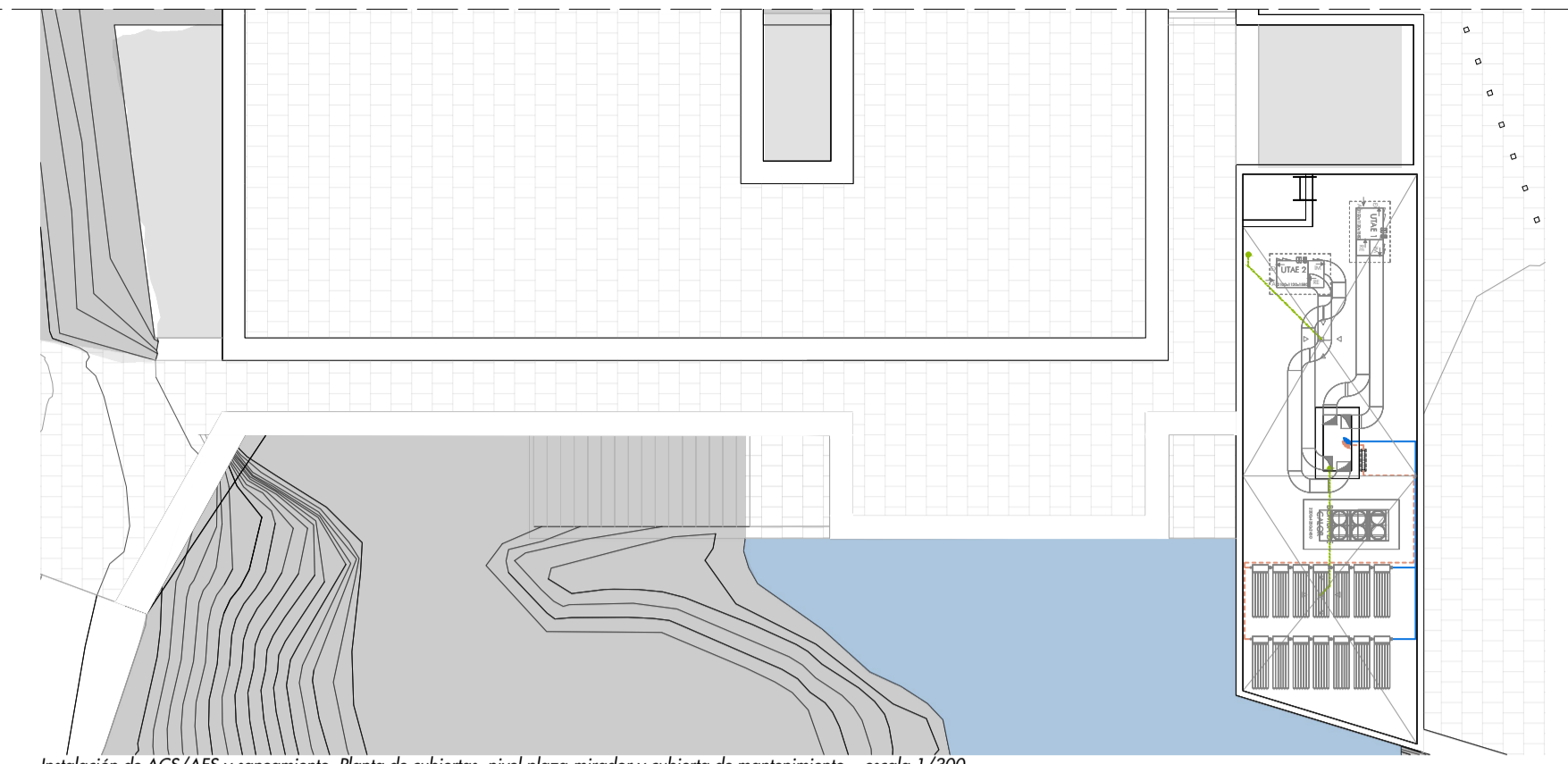
Instalación de ACS/AFS y saneamiento. Planta de cubierta, nivel plaza-mirador y cubierta de mantenimiento... escala 1/300
