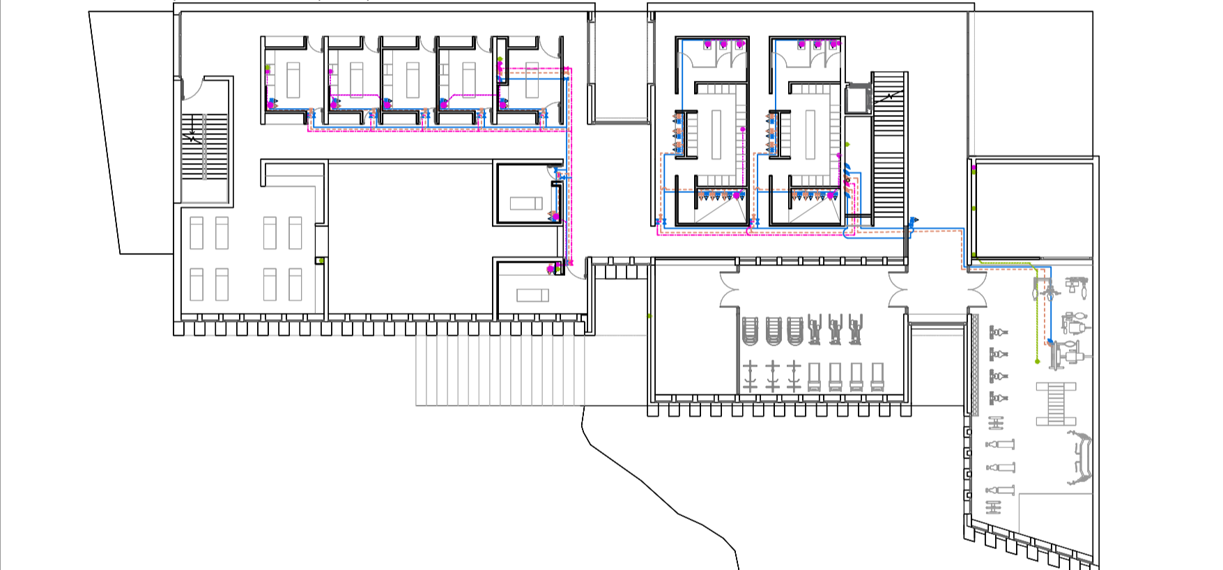
Instalación de ACS/AFS y saneamiento. Planta menos uno, nivel seco... escala 1/300
