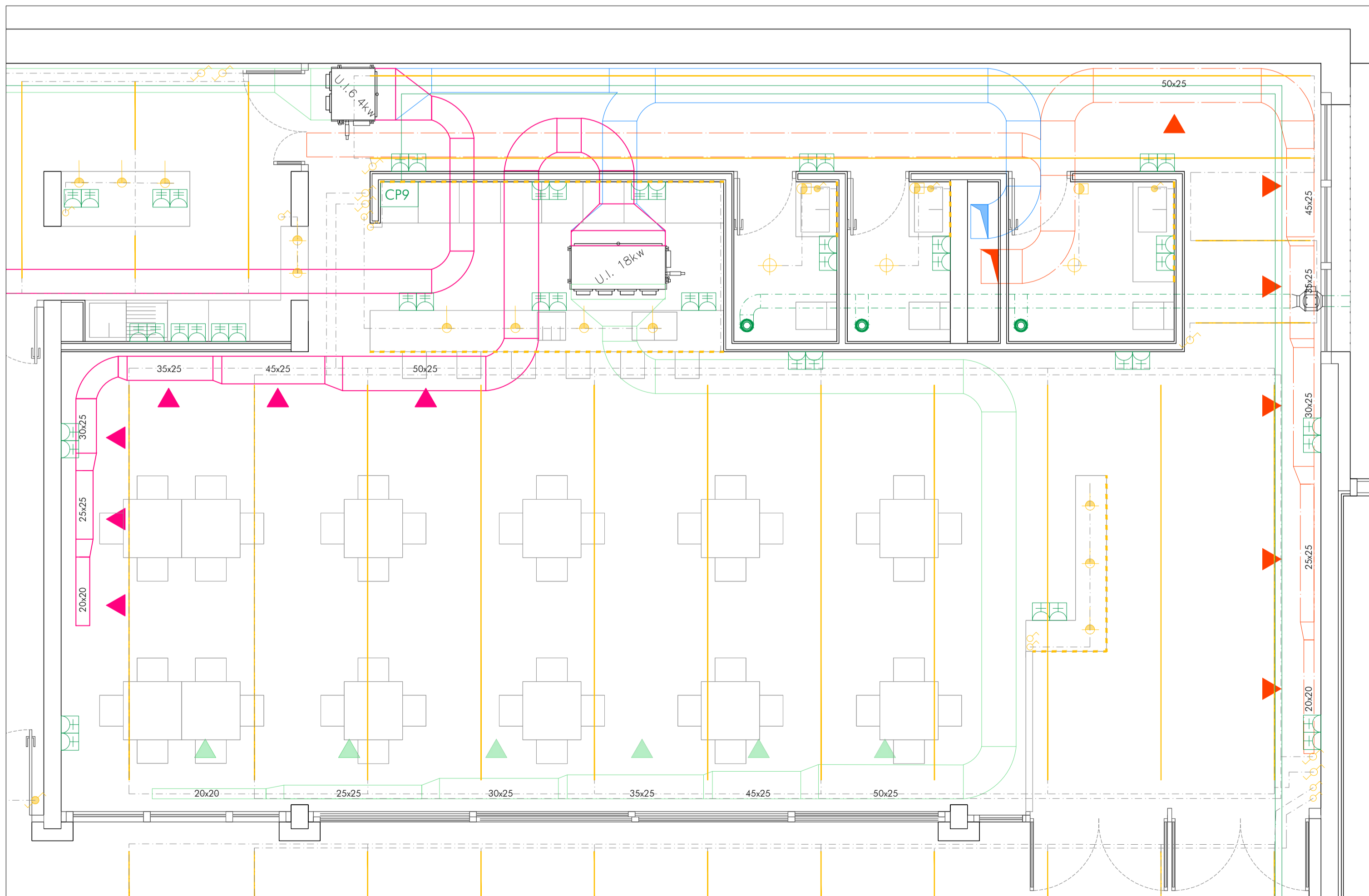
Restaurante - cafetería en planta baja, instalación de climatización-ventilación y electrotecnia... escala 1/50
