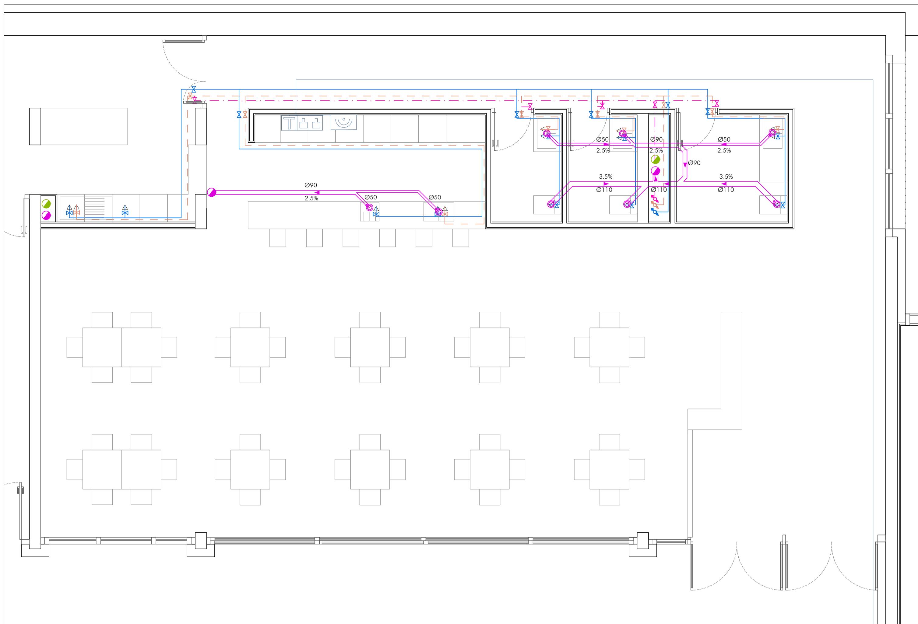
Restaurante - cafetería en planta baja, instalación de ACS/AFS, saneamiento y telecomunicaciones... escala 1/50
