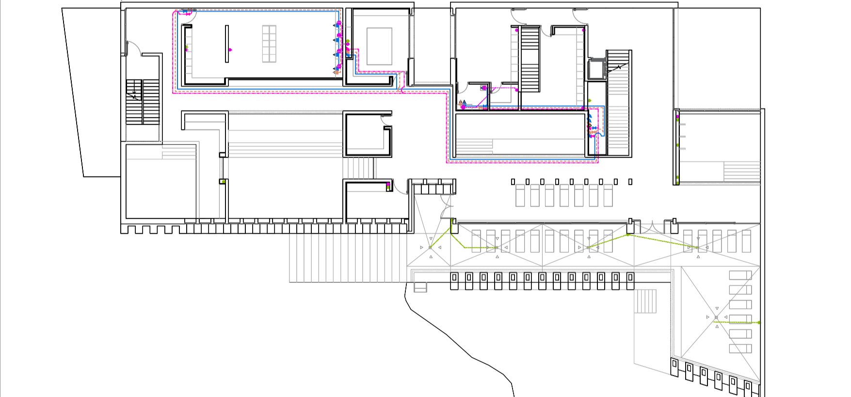
Instalación de ACS/AFS y saneamiento. Planta menos dos, nivel húmedo... escala 1/300
