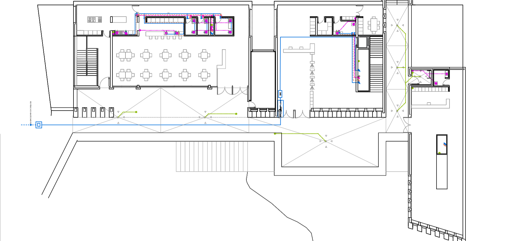
Instalación de ACS/AFS y saneamiento. Planta baja, nivel público... escala 1/300
