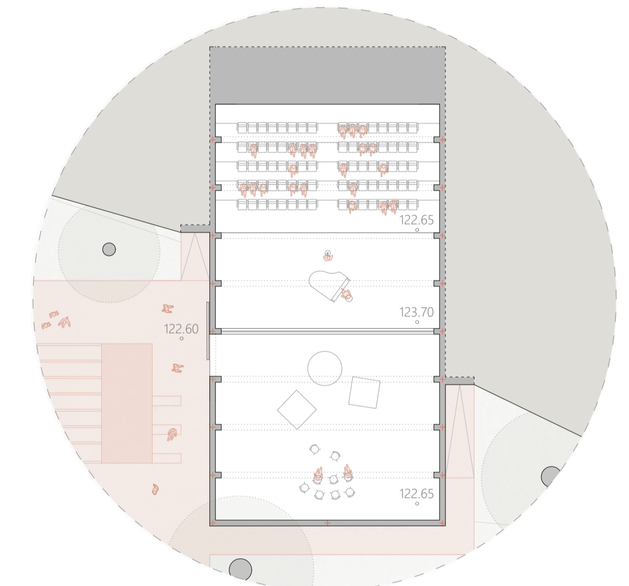
Sala expositiva +122.65
