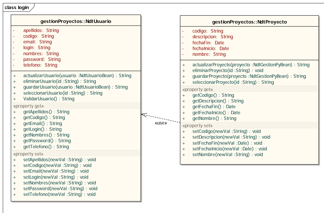
Figura 6. Diagrama de clases básico.
