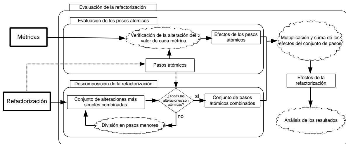
Figura 4. Proceso de evaluación.
