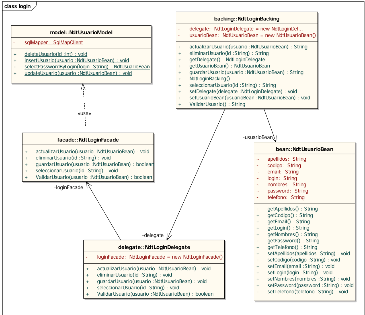
Figura 9 Diagrama de clases – Login.
