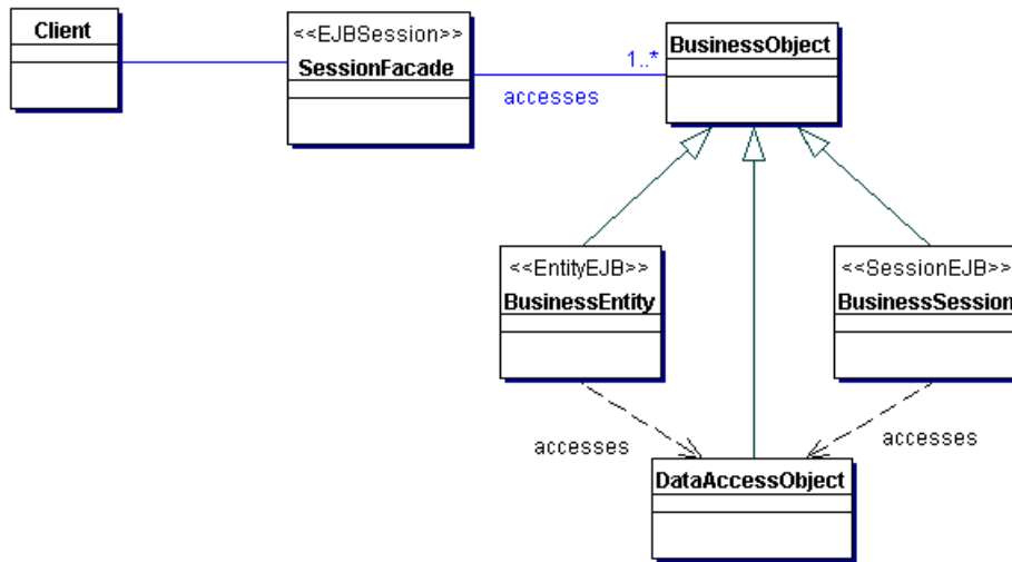
Figura 2. Estructura Session Facade.
