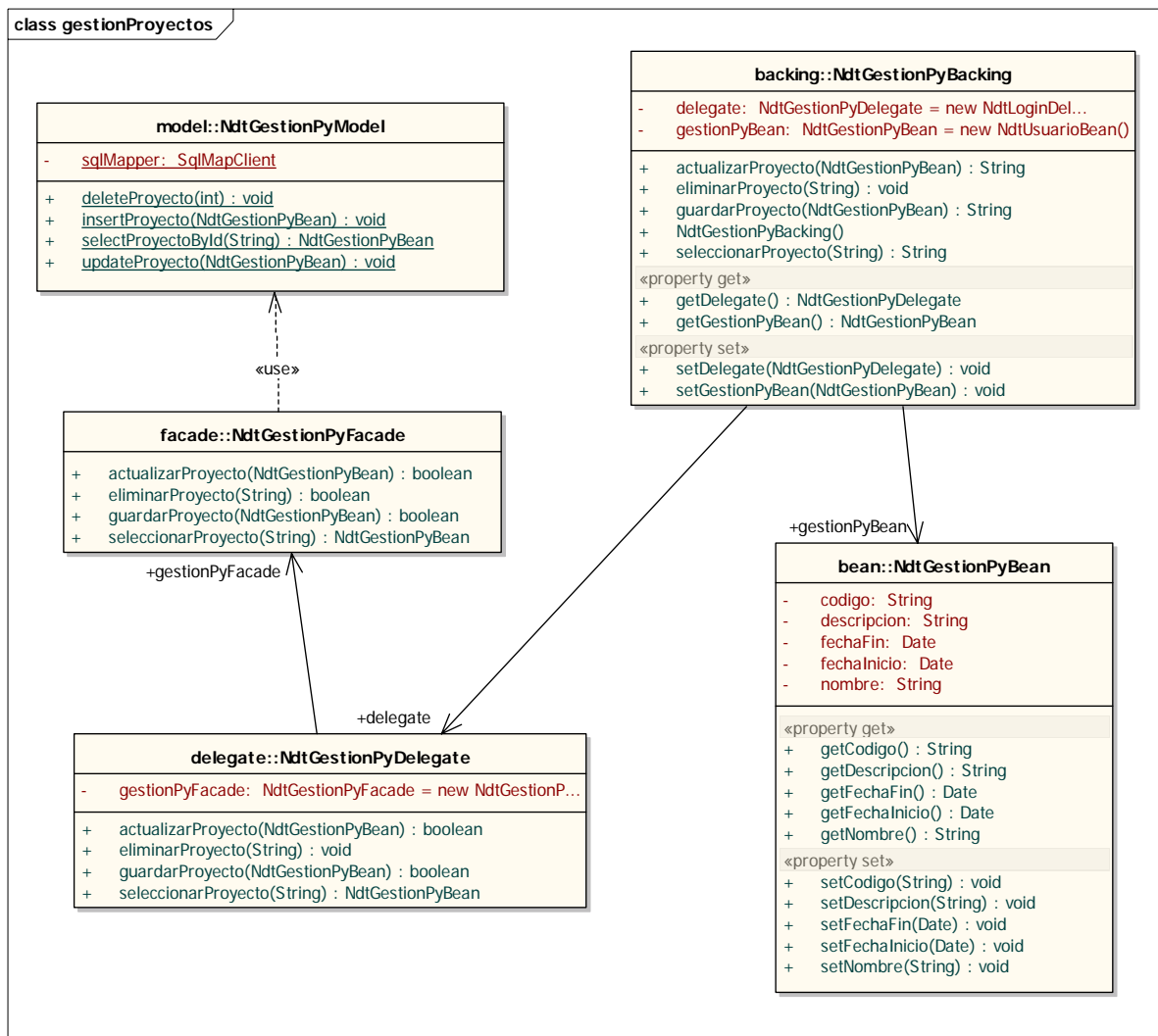
Figura 8. Diagrama de clases – Gestión de proyectos.
