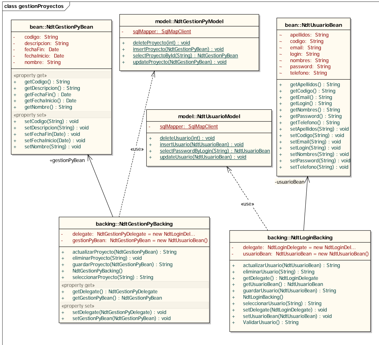
Figura 7. Diagrama de clases – Gestión de proyectos.
