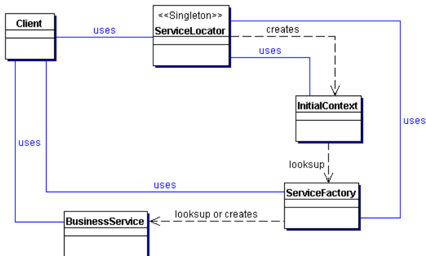
Figura 3. Estructura Service Locator.
