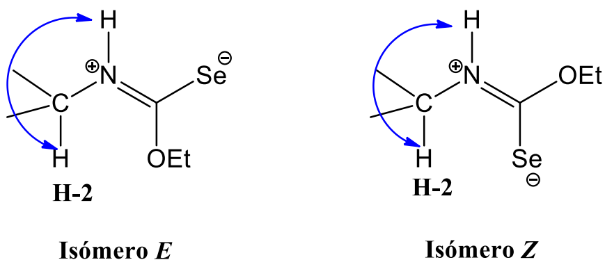
Figura 3.28. Confórmeros E/Z
