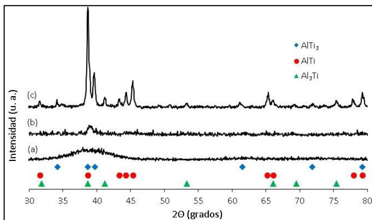
Figura 3. XRD (a) del polvo molido durante 75 hora, (b) del compacto SRE (7kA y 40s) y (c) del compacto SRE recocido a 850°C.
