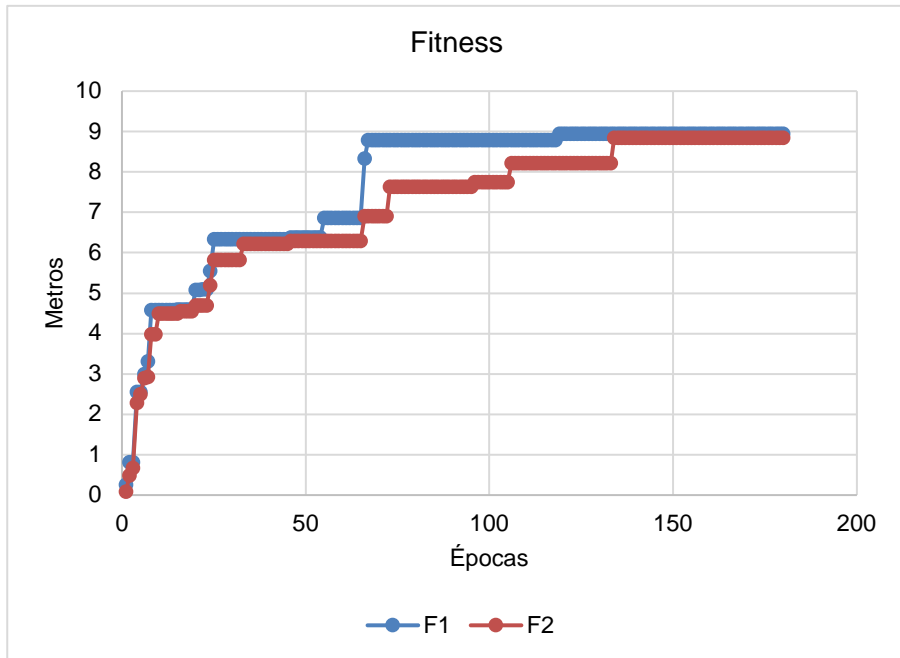
Figura 2. Evolución Fitness.
