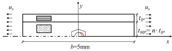
Figura 2.- Modelo BEM multiescala de un laminado [0,90n]s.
