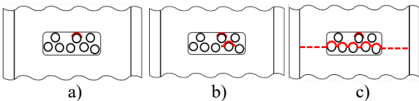
Figura 1. a) Aparecen despegues aislados. b) Se produce el kinking de la grieta de interfase. c) Se genera la grieta transversal.
