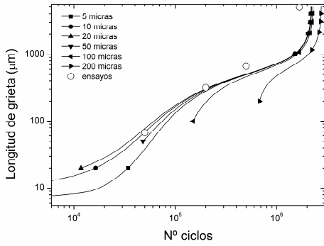
Figura 3. Evolución de la grieta en los ensayos con \sigma = 45 \text{ MPa} , Q = 210 \text{ N} y N = 420 \text{ N} .
