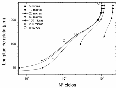
Figura 4. Evolución de la grieta en los ensayos con \sigma = 60 \text{ MPa} , Q = 120 \text{ N} y N = 240 \text{ N} .
