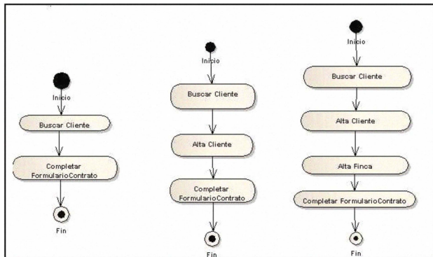
Figura 3: Casos de Pruebas para el ejemplo
