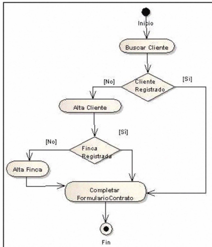
Figura 2: Requisito Funcional para el ejemplo
