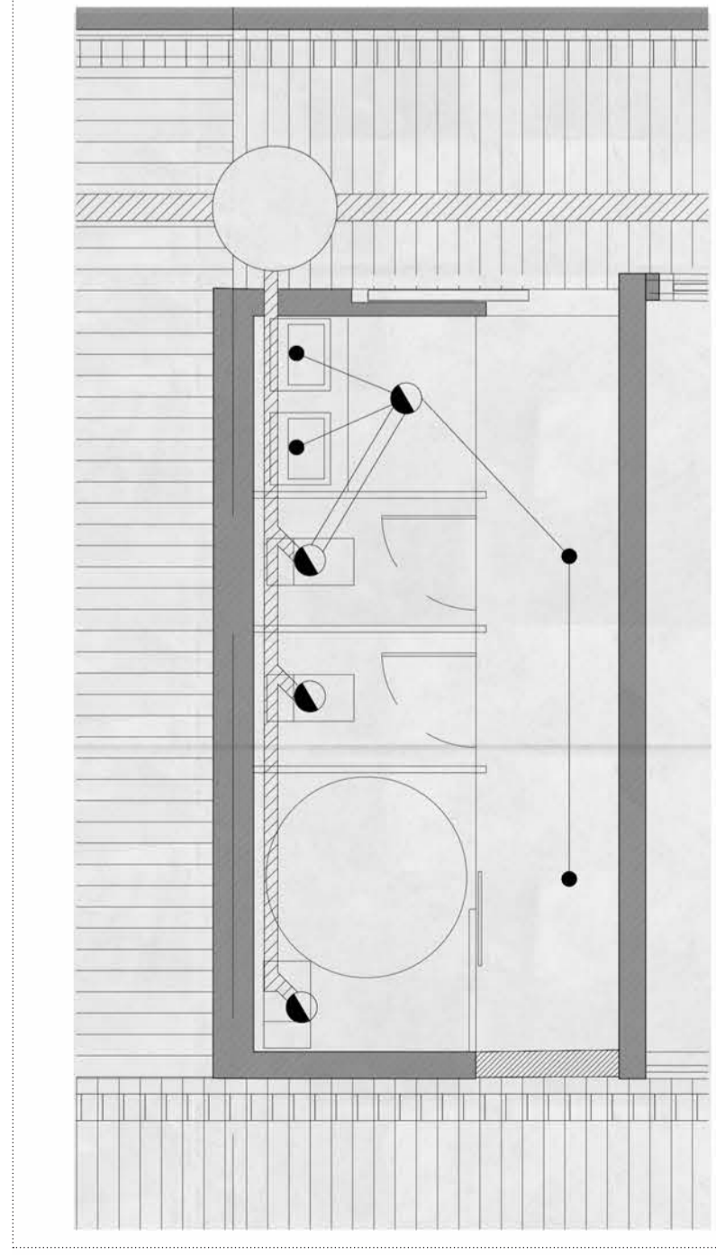
DETALLE NÚCLEO HÚMEDO. E: 1/50
