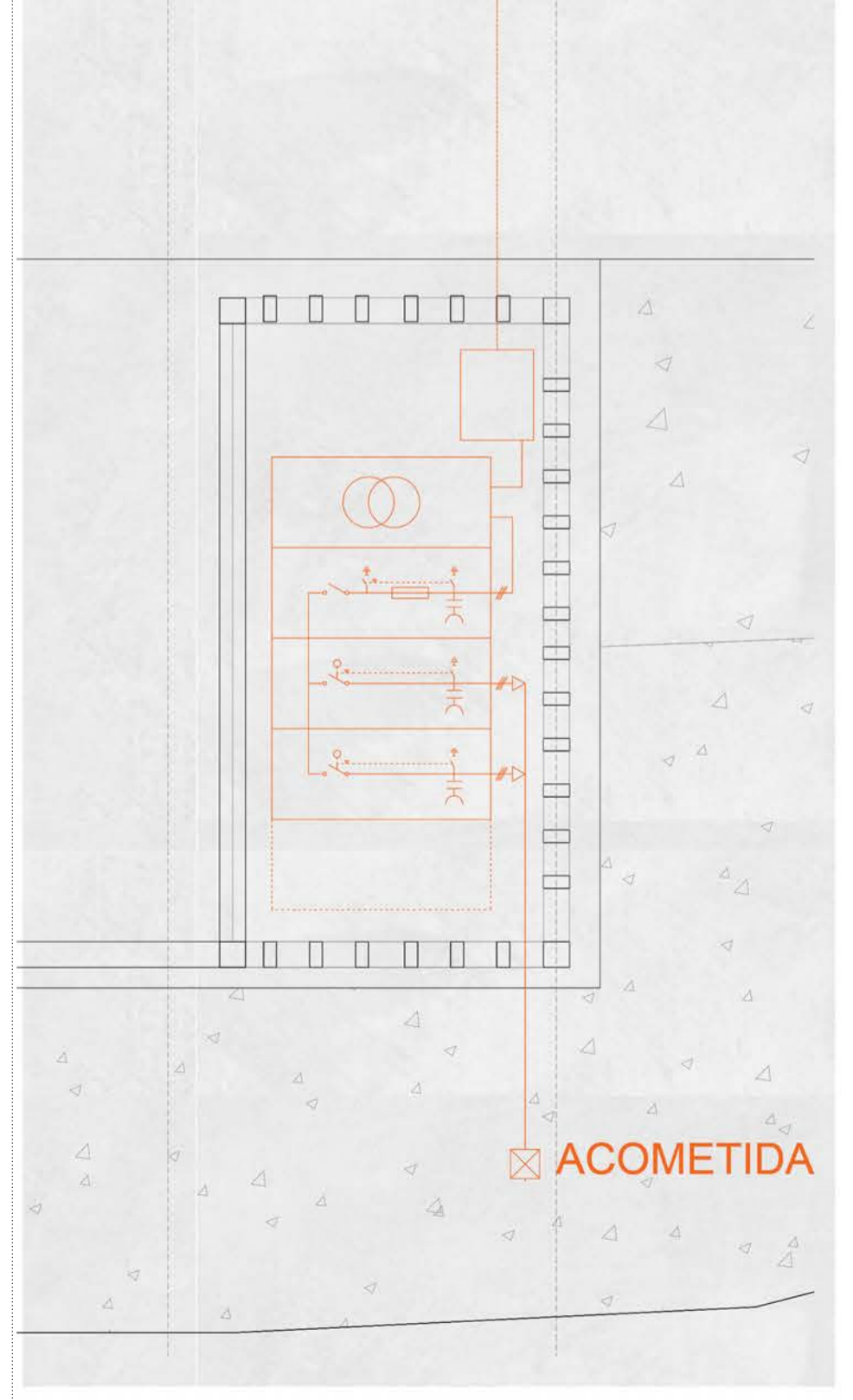
DETALLE DEL EQUIPO TRANSFORMADOR E. 1/75
