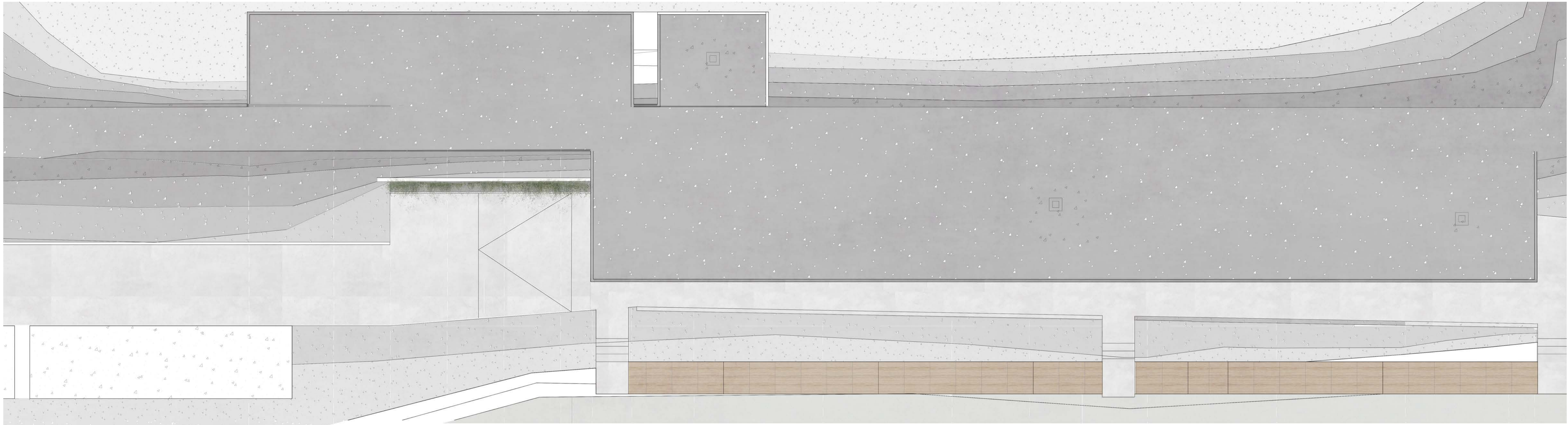
PLANTA CUBIERTA E. 1/150 0m 10m
