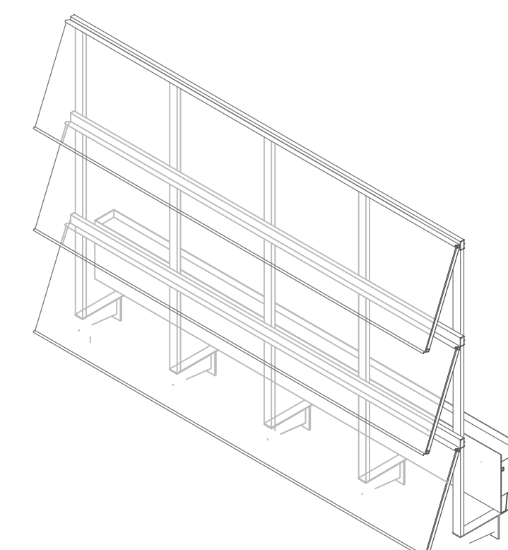
DESPIECE DE LAMAS DE POLICARBONATO Y SUBESTRUCTURA
