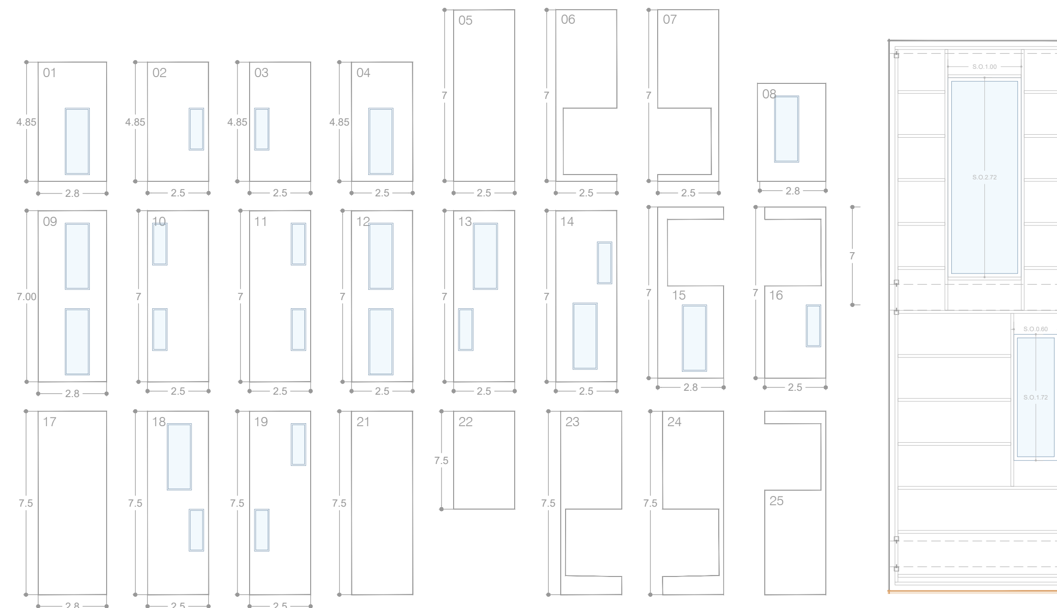
DESPIECE DE PANELES GRC Stud Frame
