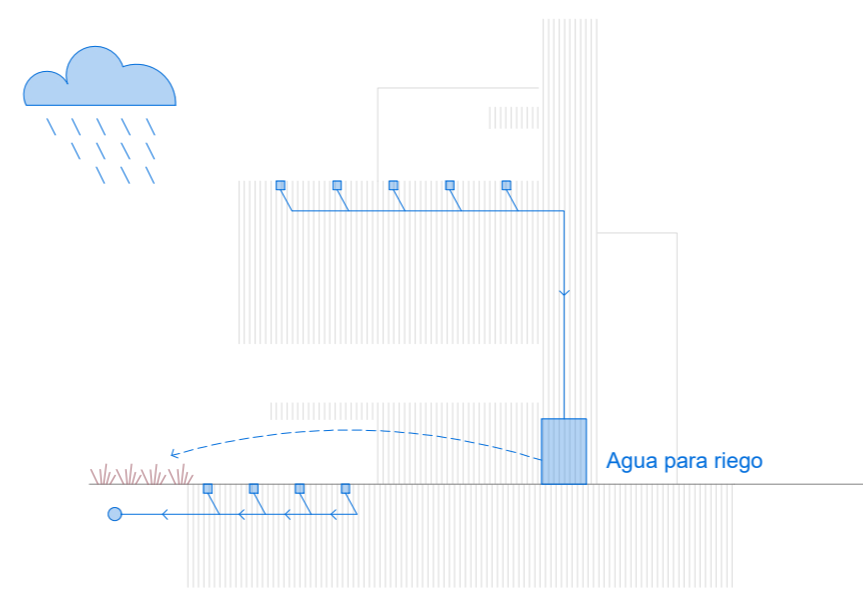
CICLO DEL AGUA Pluviales
