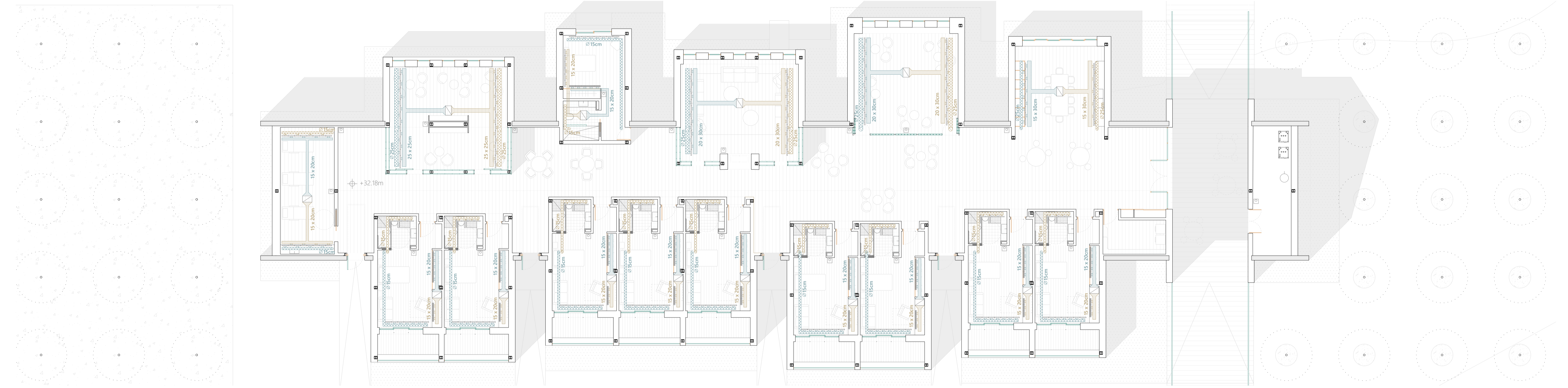
PLANTA COTA +0,18m. ESCALA 1:125
