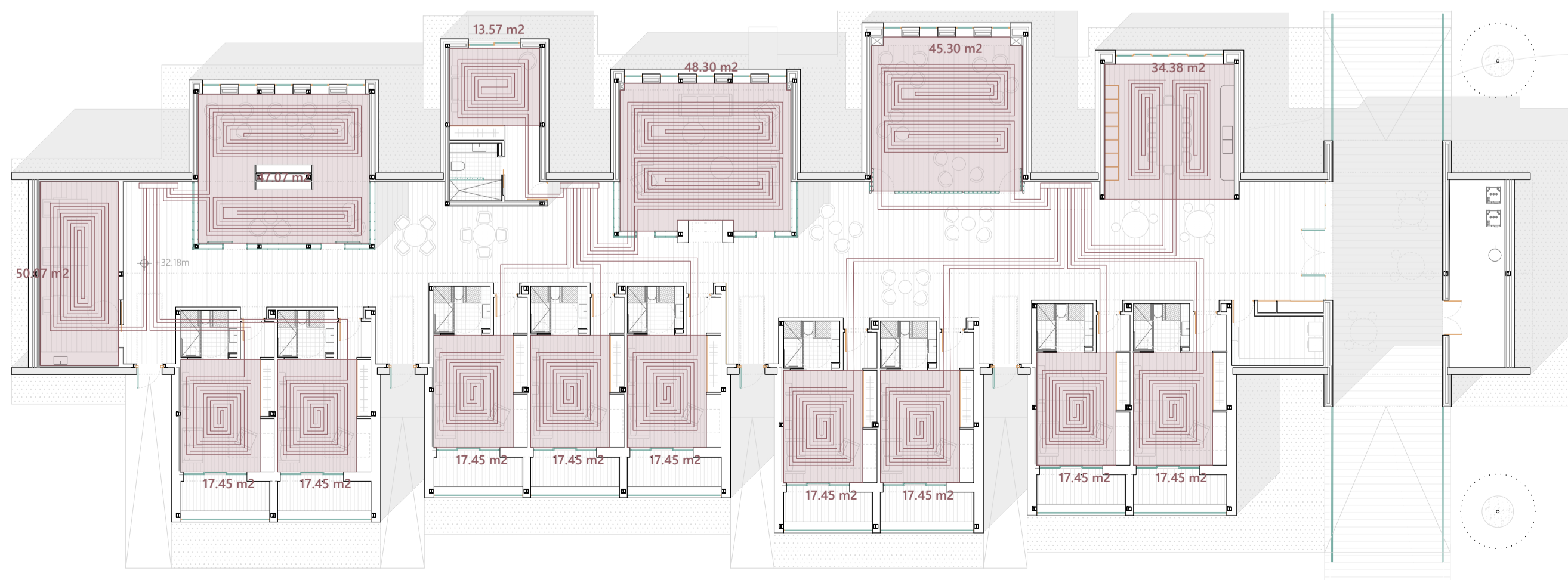
PLANTA COTA +0,18m. ESCALA 1:125
