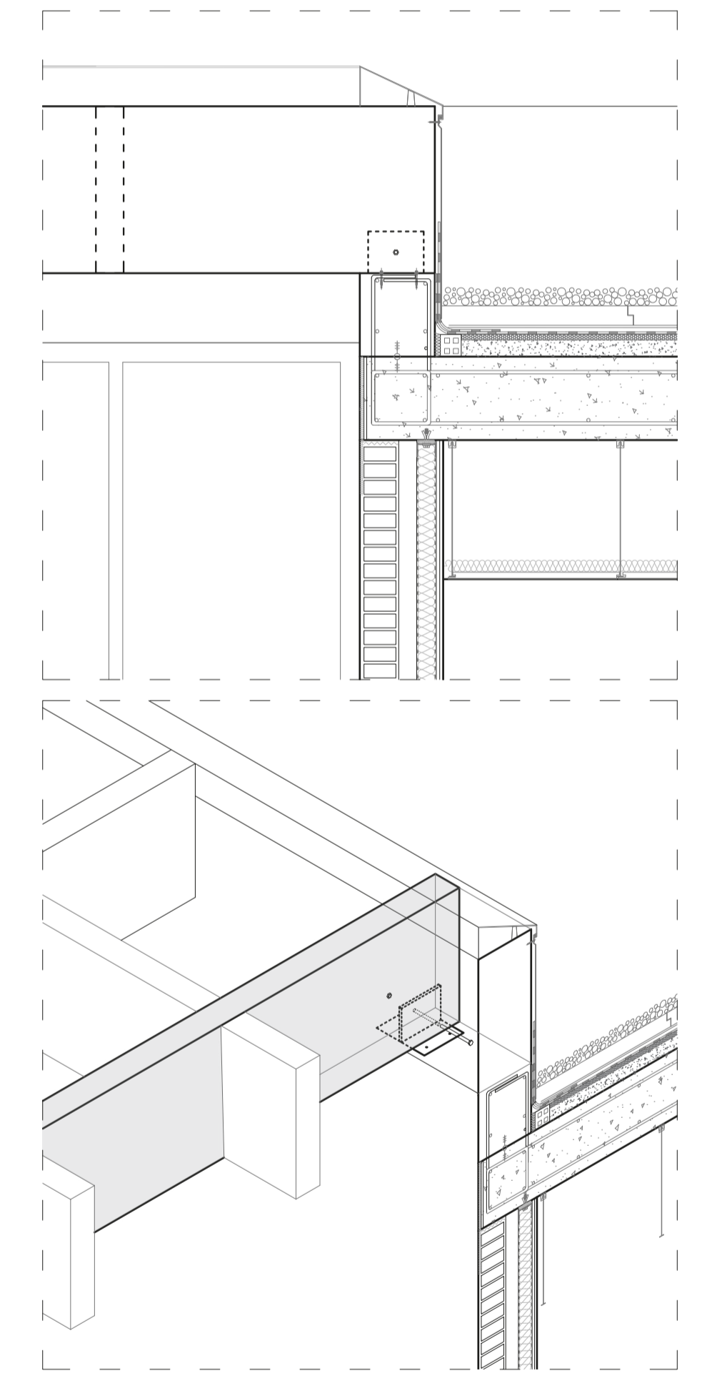
ENCUENTRO EMPARRILLADO Y FORJADO 1:20
