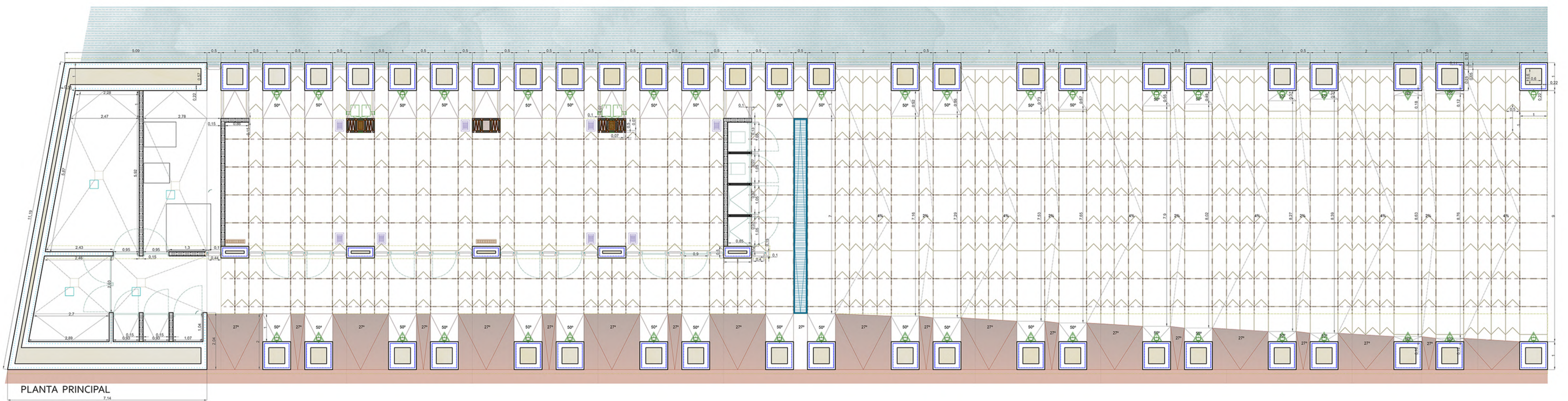
PLANTA PRINCIPAL
