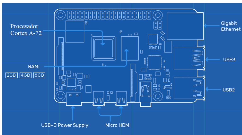
Ilustración 2-8: Raspberry Pi 4B
