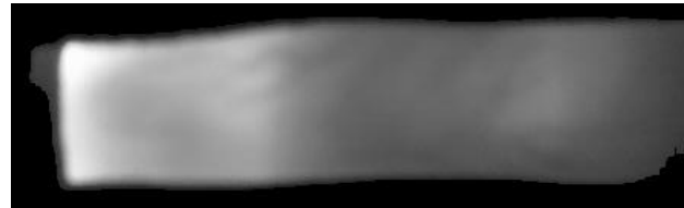
Ilustración 3-3: Dedo umbralizado
