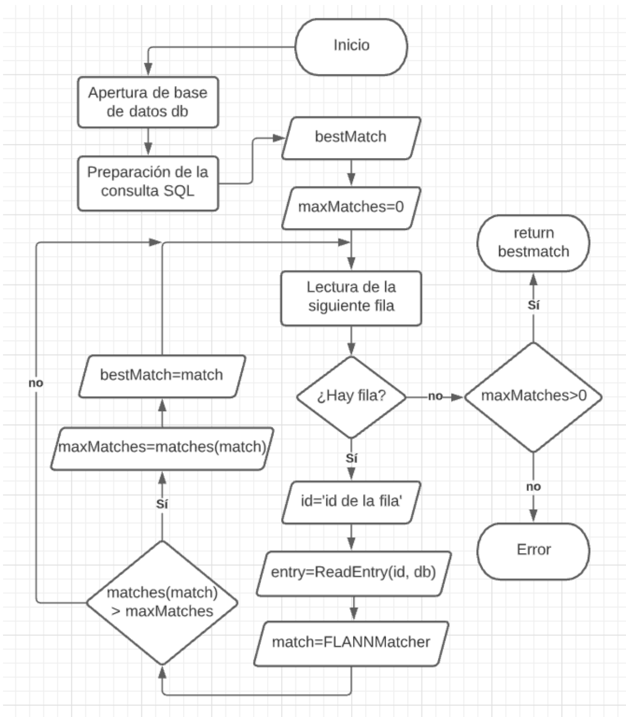
Ilustración 3-17: Diagrama de flujo de función de búsqueda de mejor coincidencia
