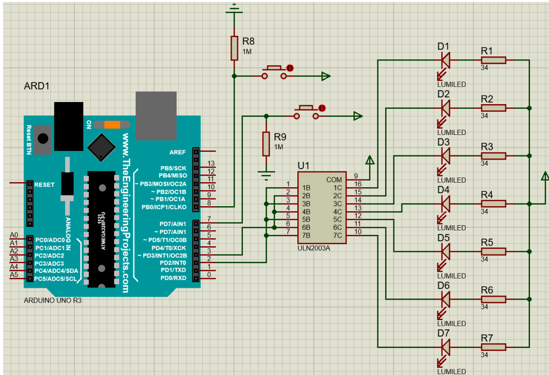
Ilustración 2-7: Montaje de prueba con Arduino
