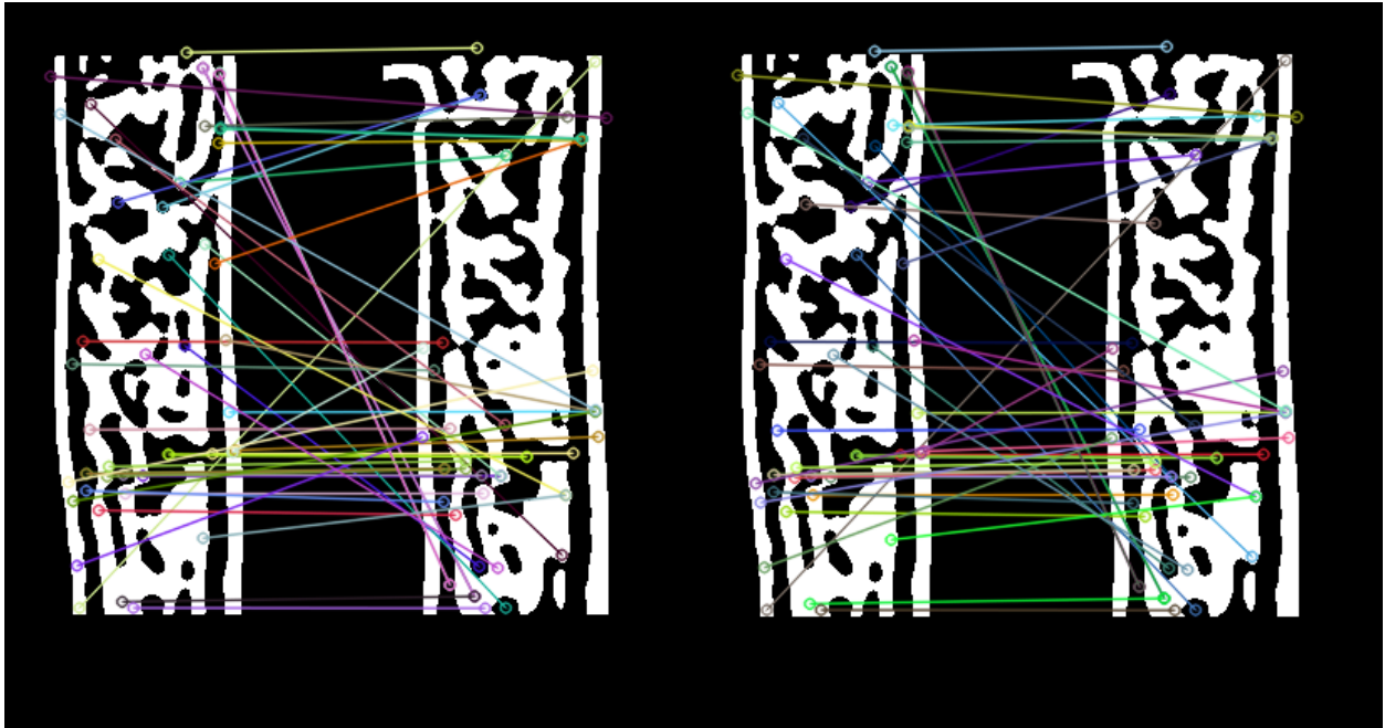
Ilustración 3-14: Correspondencia SIFT sin descartar por inclinación
