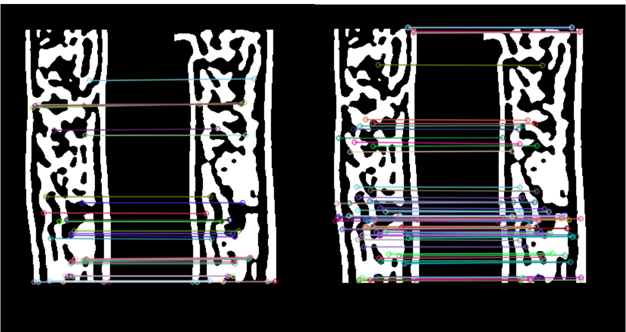
Ilustración 3-8: Correspondencia ORB
