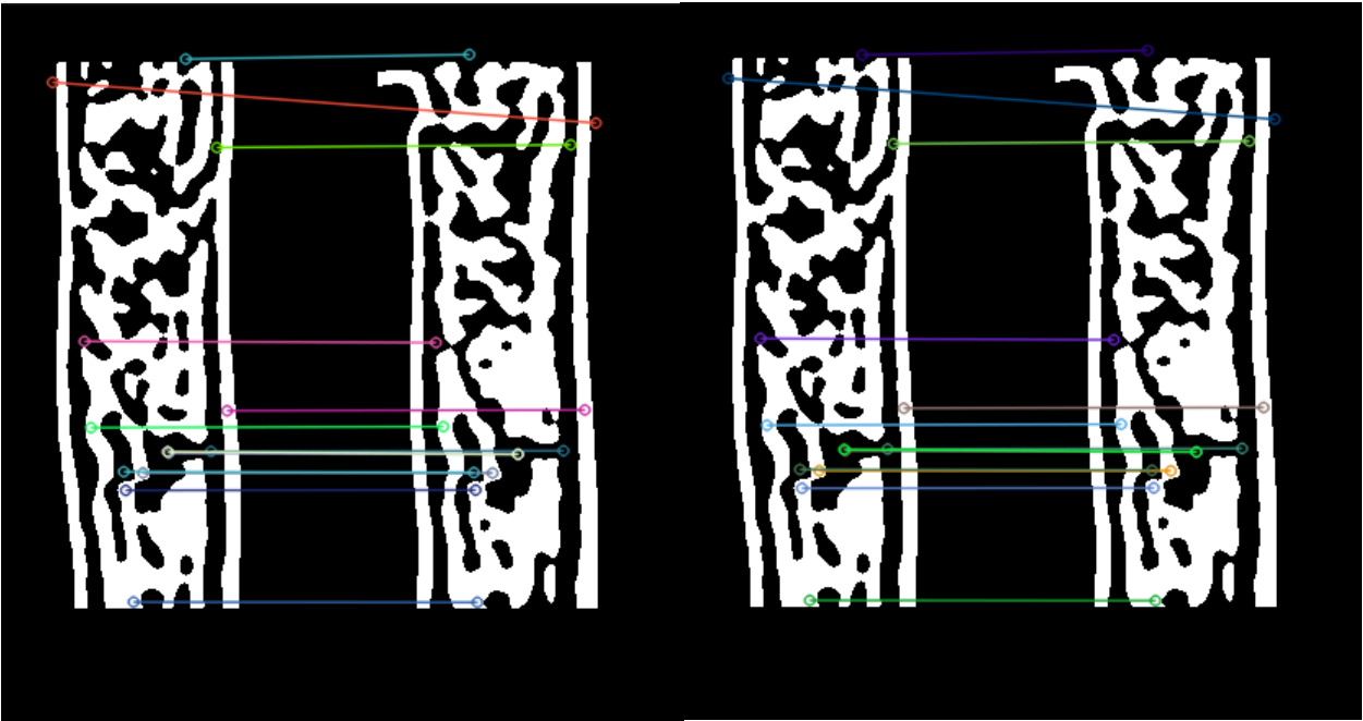
Ilustración 3-11: Correspondencia SIFT
