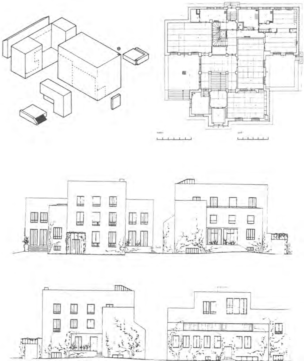
La Kundmannngasse, composición volumétrica, planta y alzados
