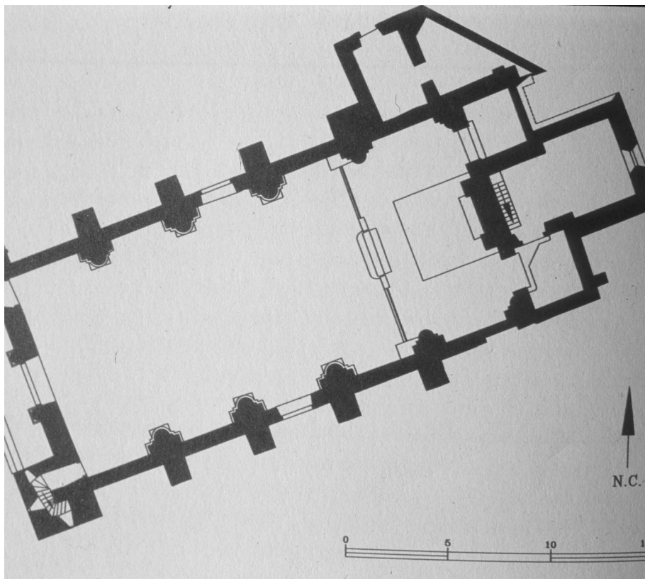
Figura 8. Marmelar. Iglesia de la Vera Cruz. Planta (A. Pagará).
