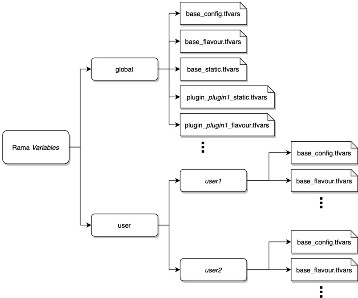
Figura 10 Estructura de directorios y ficheros de la rama de variables
