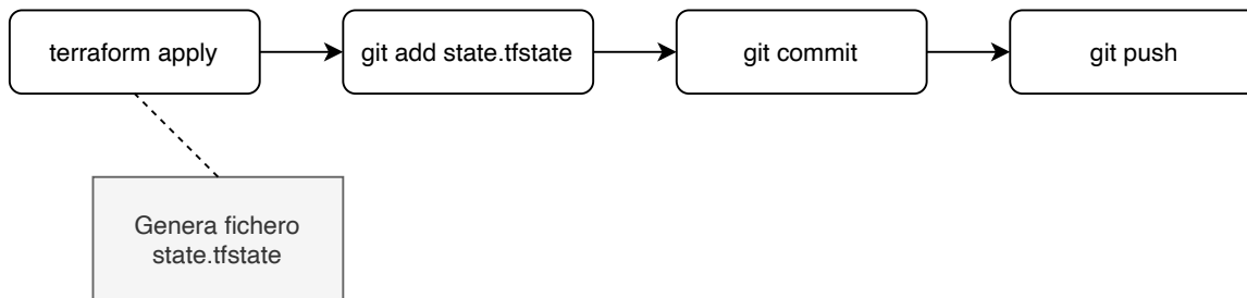
Figura 7 Diagrama de flujo con los comandos para el almacenado en git del estado
