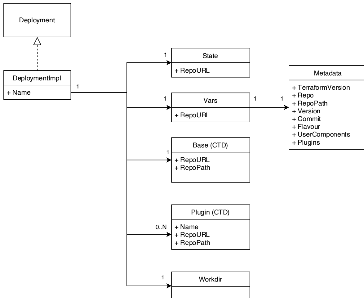
Figura 11 Diagrama de clases del paquete Deployment
