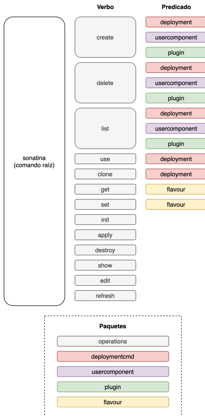
Figura 16 Subcomandos de Sonatina clasificados por paquetes
