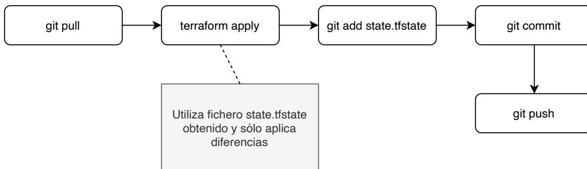
Figura 8 Diagrama de flujo con los comandos para trabajar colaborativamente con el estado
