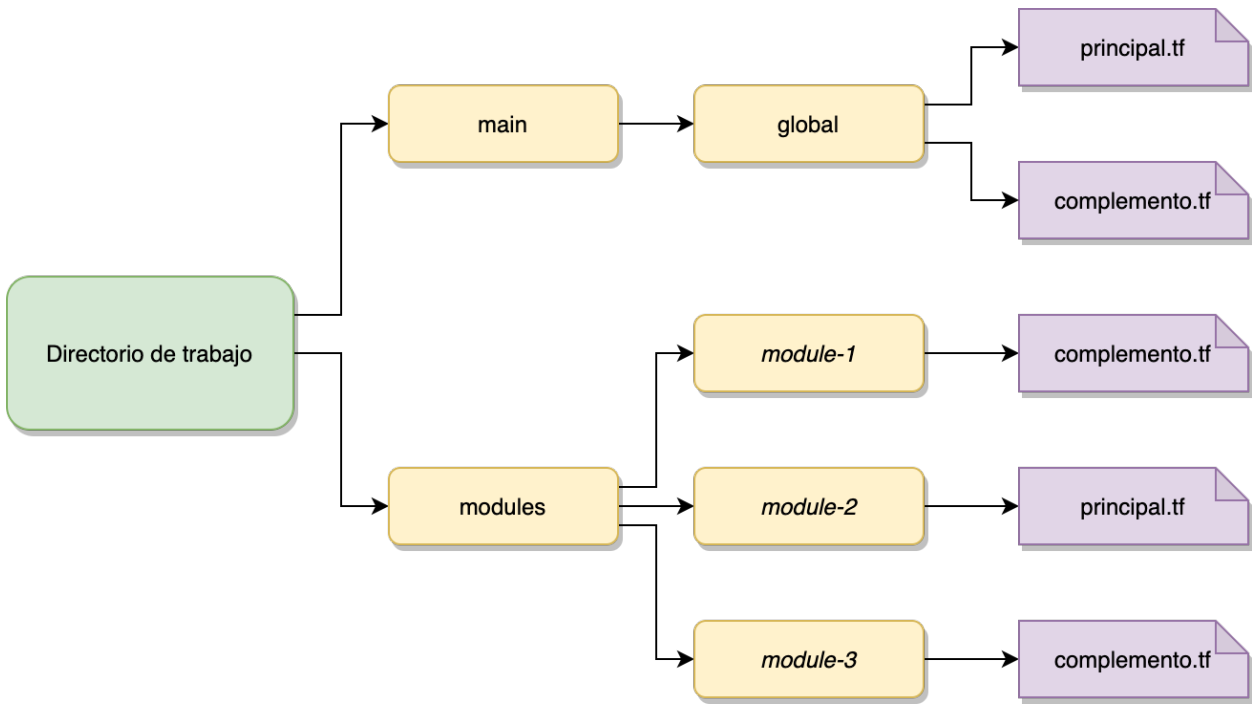
Figura 5 Directorio de trabajo de ejemplo para el componente global
