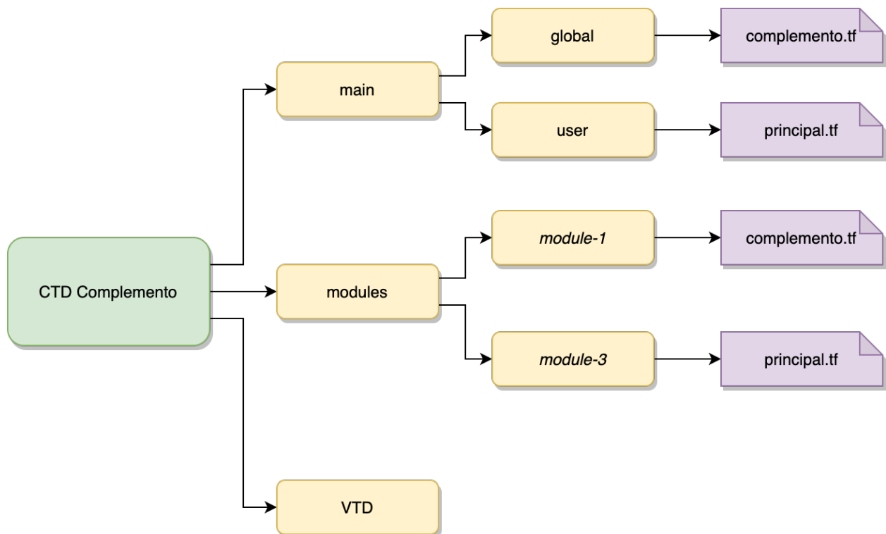
Figura 4 CTD del complemento de ejemplo
