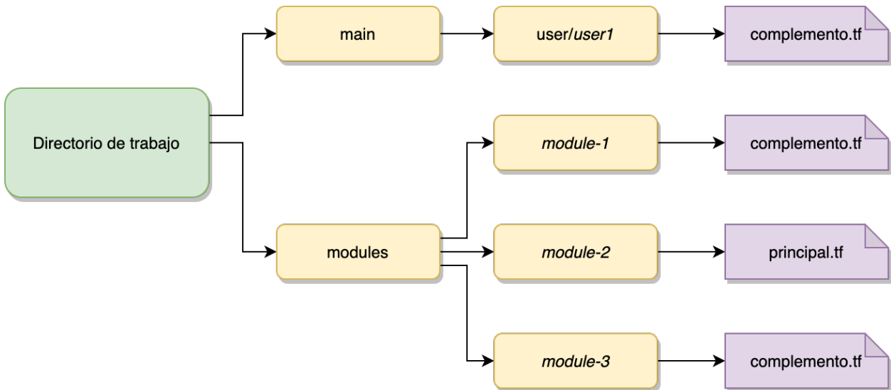
Figura 6 Directorio de trabajo de ejemplo para el componente de usuario
