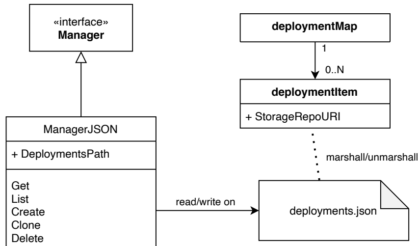
Figura 12 Diagrama de clases del componente Manager
