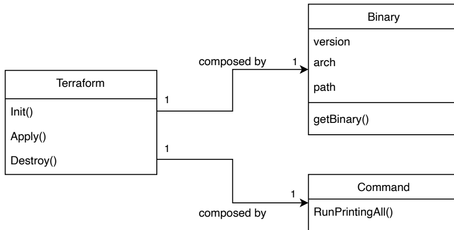
Figura 15 Diagrama de clases del paquete terraformcli
