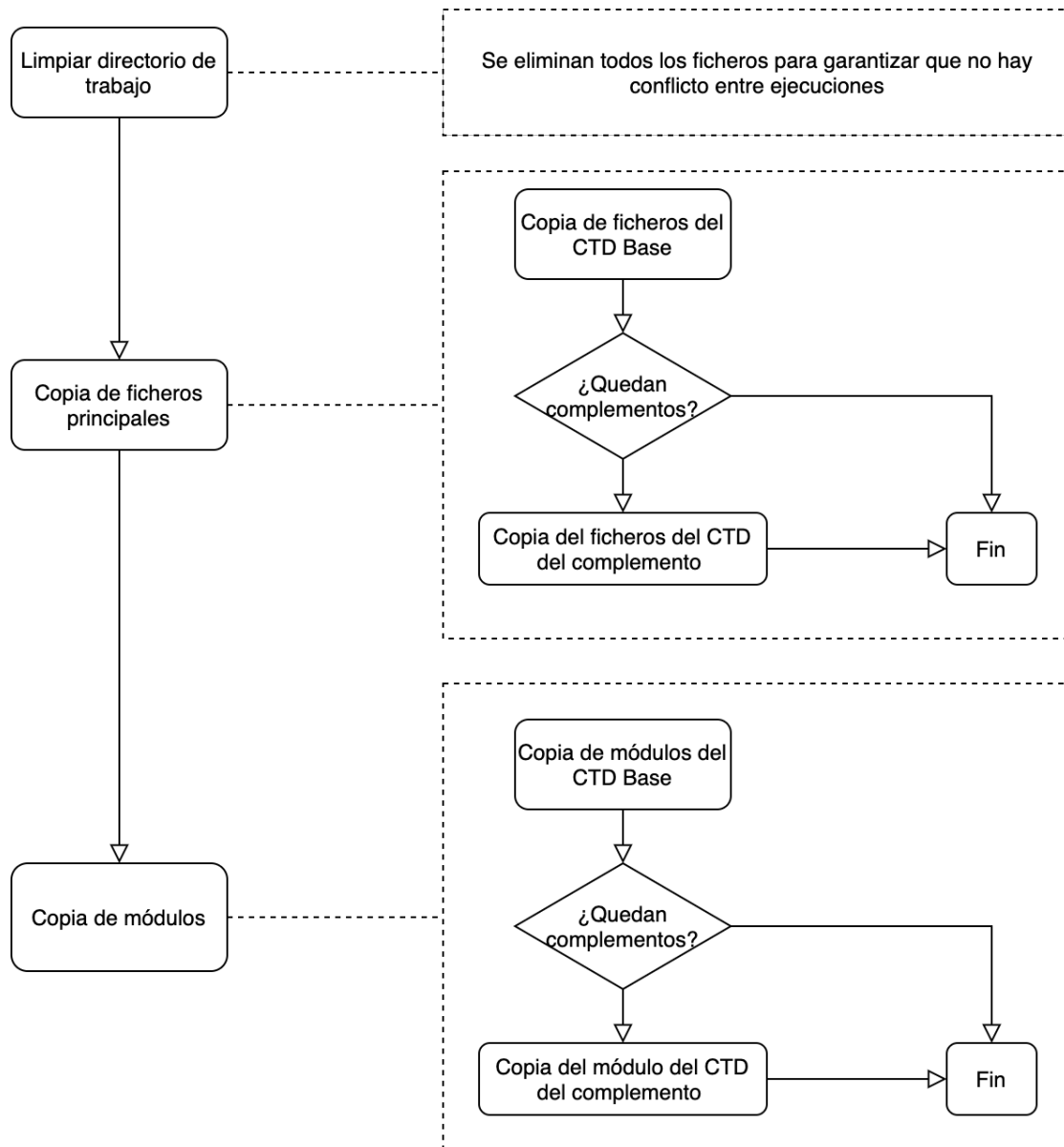
Figura 14 Diagrama de flujo de la generación del directorio de trabajo
