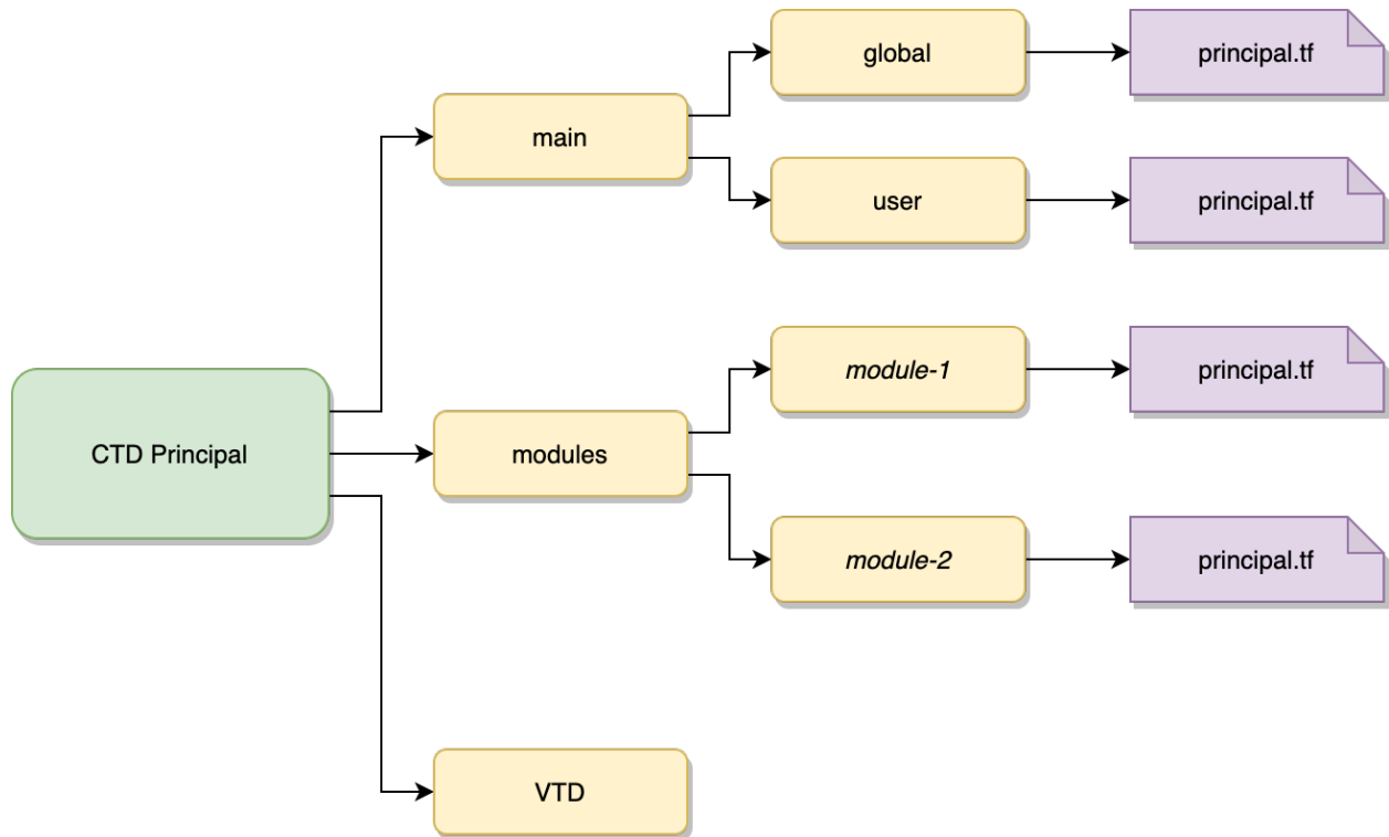
Figura 3 CTD principal de ejemplo
