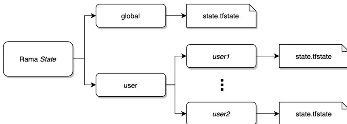
Figura 9 Estructura de directorios y ficheros de la rama de estado
