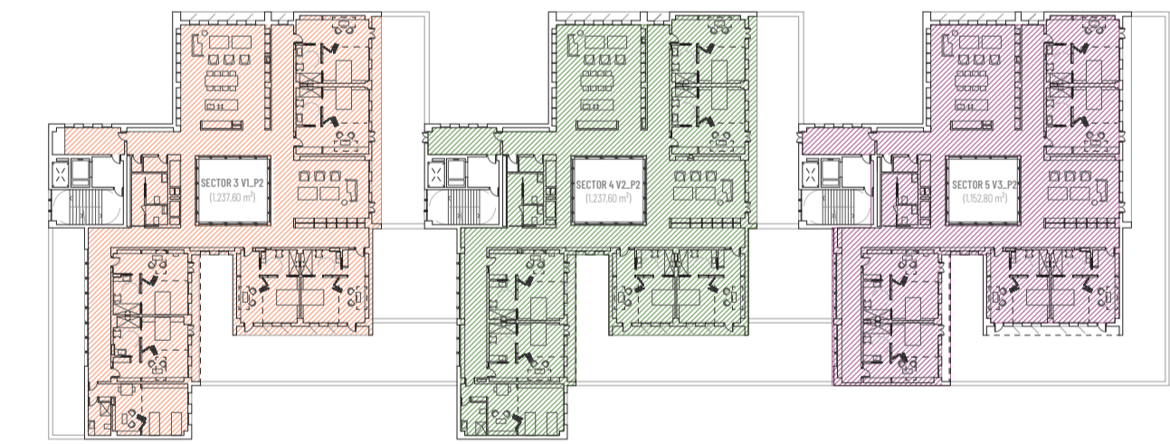
Planta segunda
