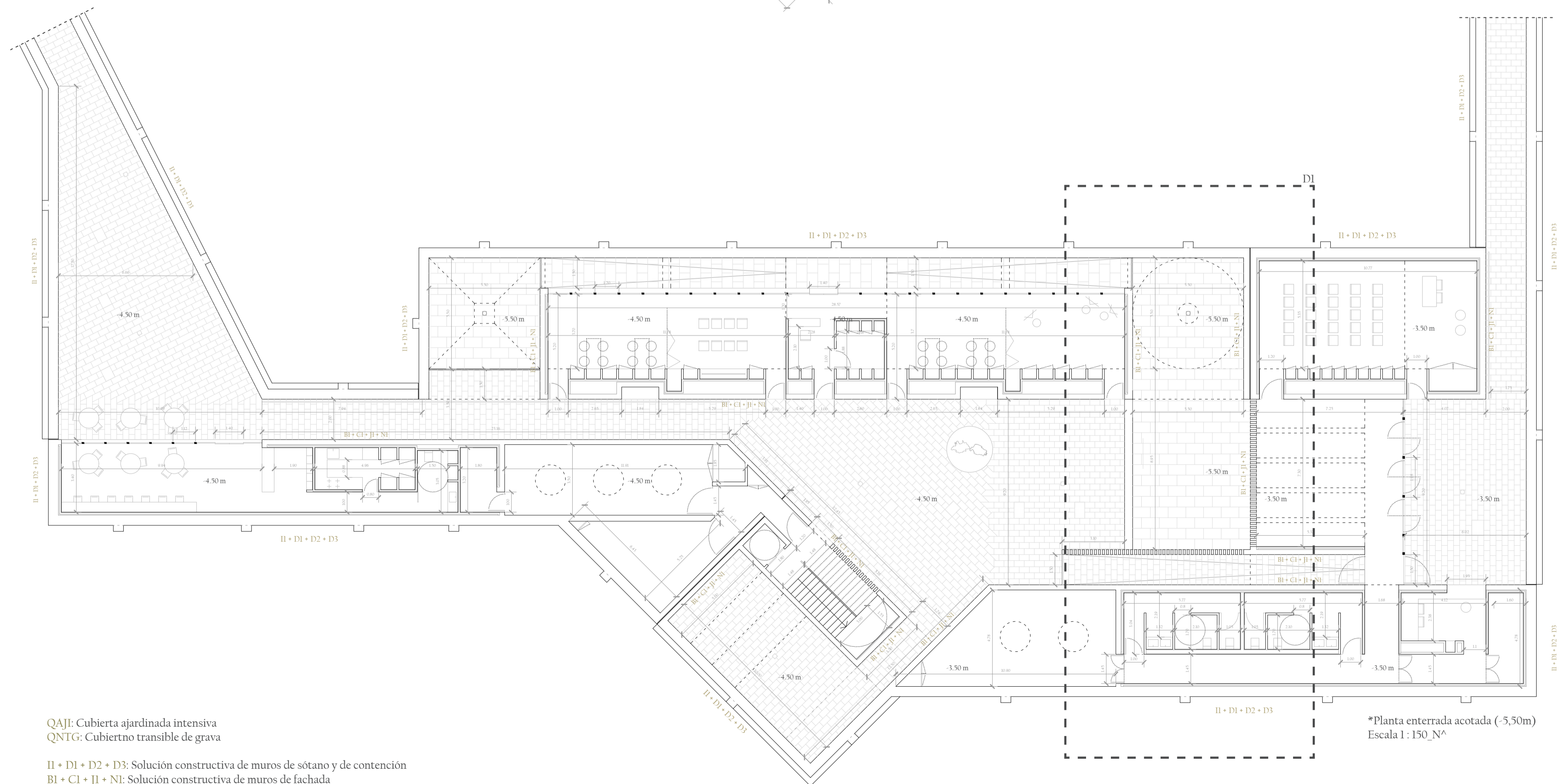
*Planta de cubierta acotada (+0,00m) Escala 1: 150_N o
