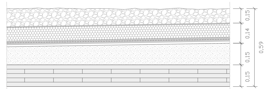
C1: CUBIERTA INVERTIDA NO TRANSITABLE CON GRAVA_E 1/15
