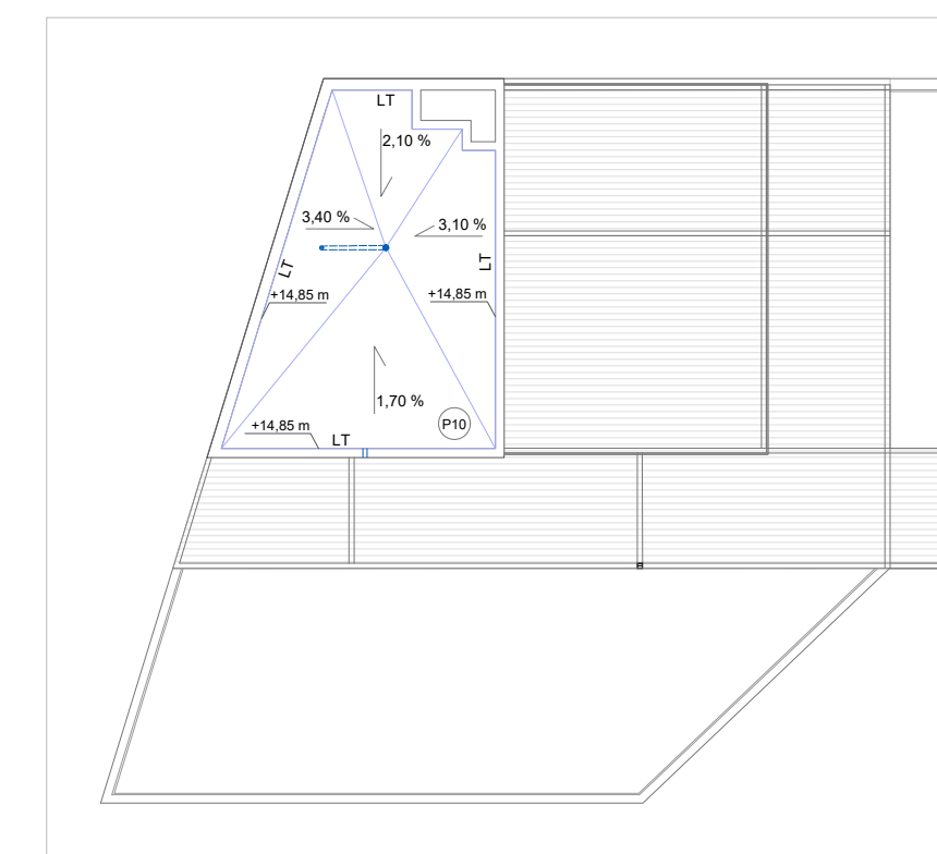
D2: CASTILLETE NÚCLEO COMUNICACIONES 3_E 1/200
