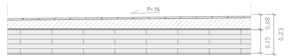
C3: FORJADO TERRAZAS VIVIENDAS CON TARIMA FLOTANTE_E 1/15
