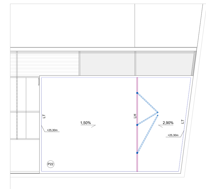
D4: CASTILLETE NÚCLEO COMUNICACIONES 2_E 1/200
