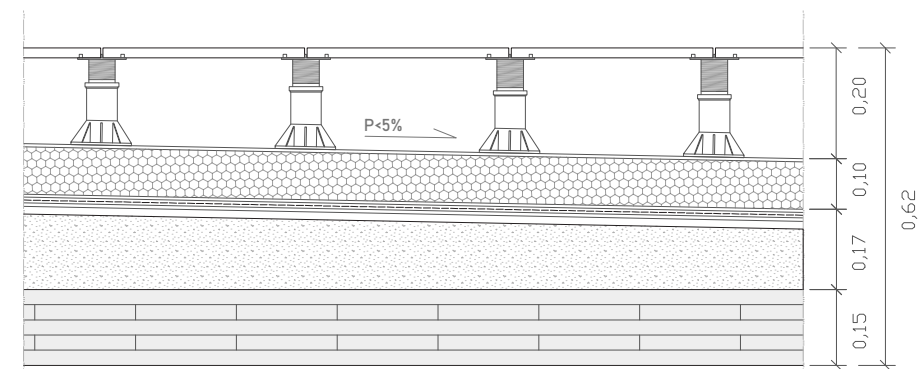
C2: CUBIERTA INVERTIDA TRANSITABLE CON PAVIMENTO FLOTANTE E 1/15
