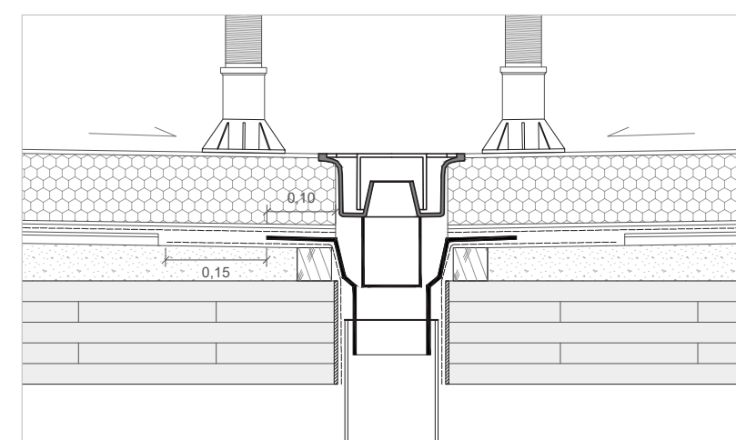
ENCUENTRO CUBIERTA TRANSITABLE Y SUMIDERO_E 1/10
