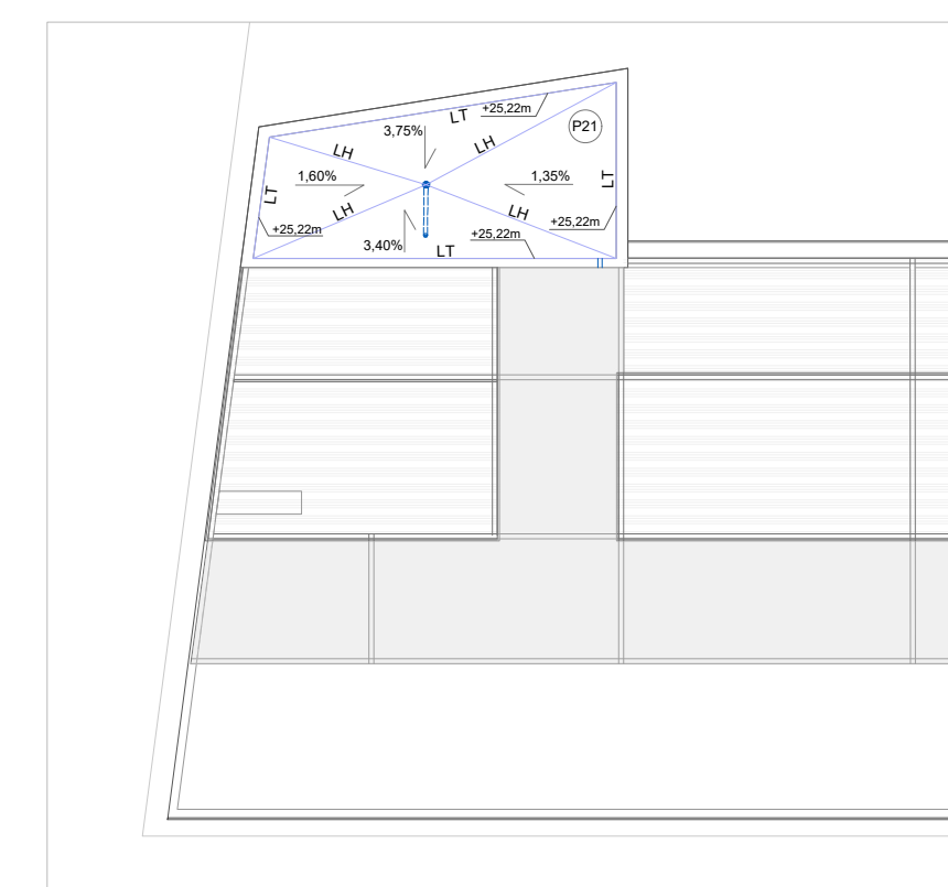
D3: CASTILLETE NÚCLEO COMUNICACIONES 1_E 1/200
