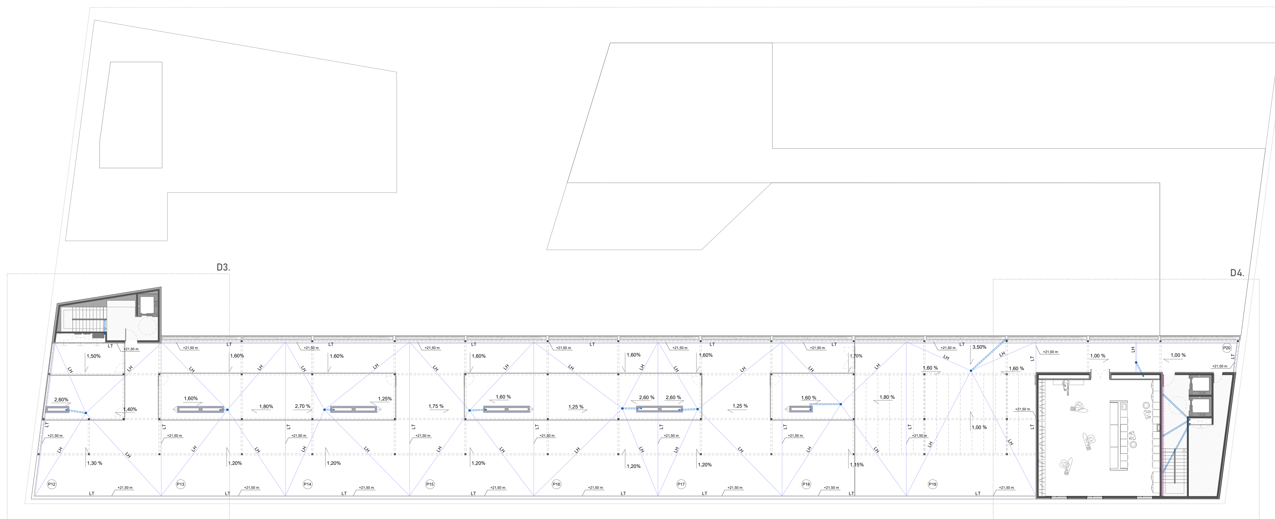
PLANTA SEXTA: EVACUACIÓN DE AGUAS PLUVIALES_E 1/200
