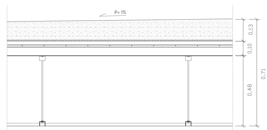
C4: FORJADO GALERÍA CON HORMIGÓN FRATASADO_E 1/15
