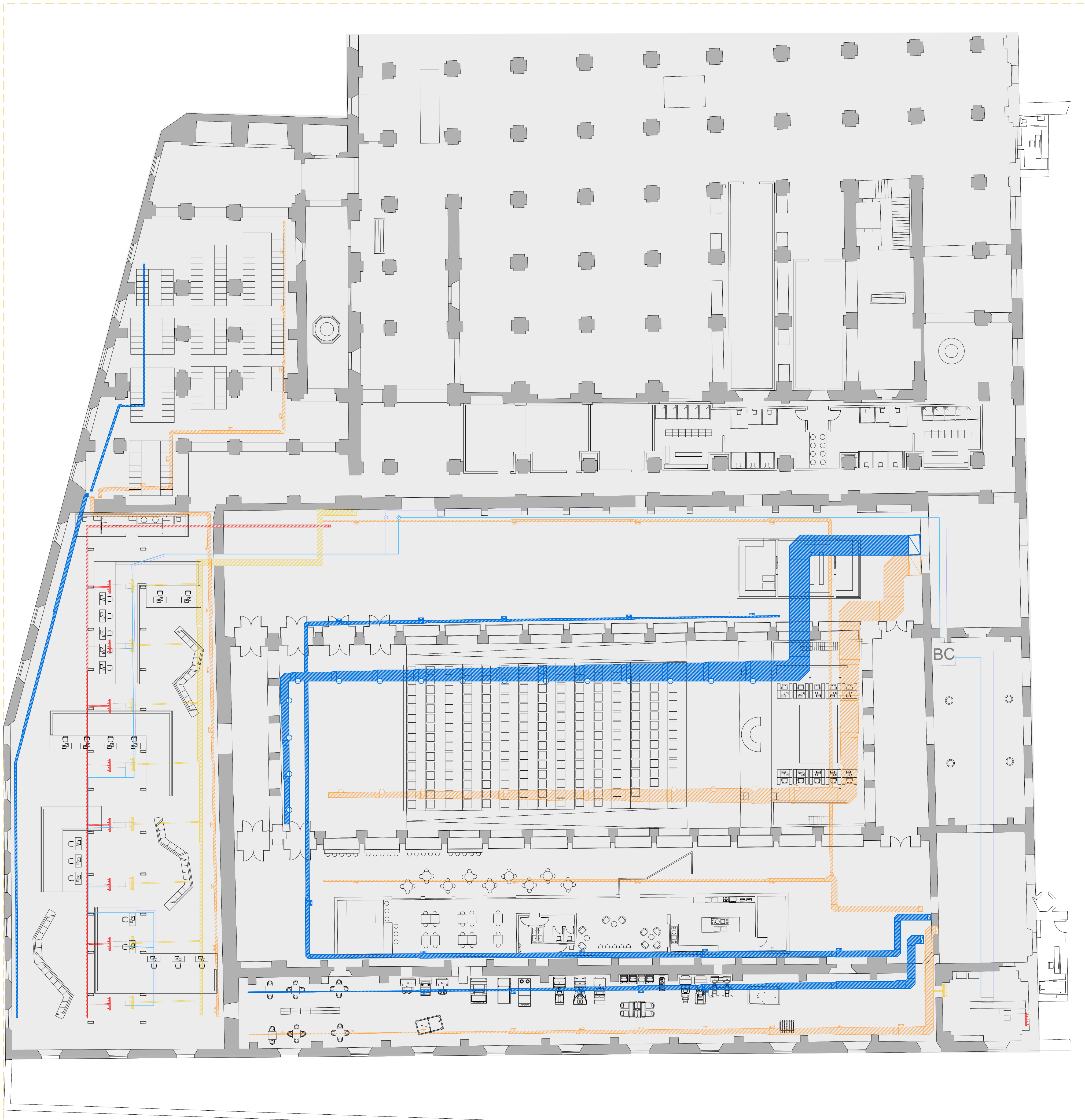
- Planta baja. -
