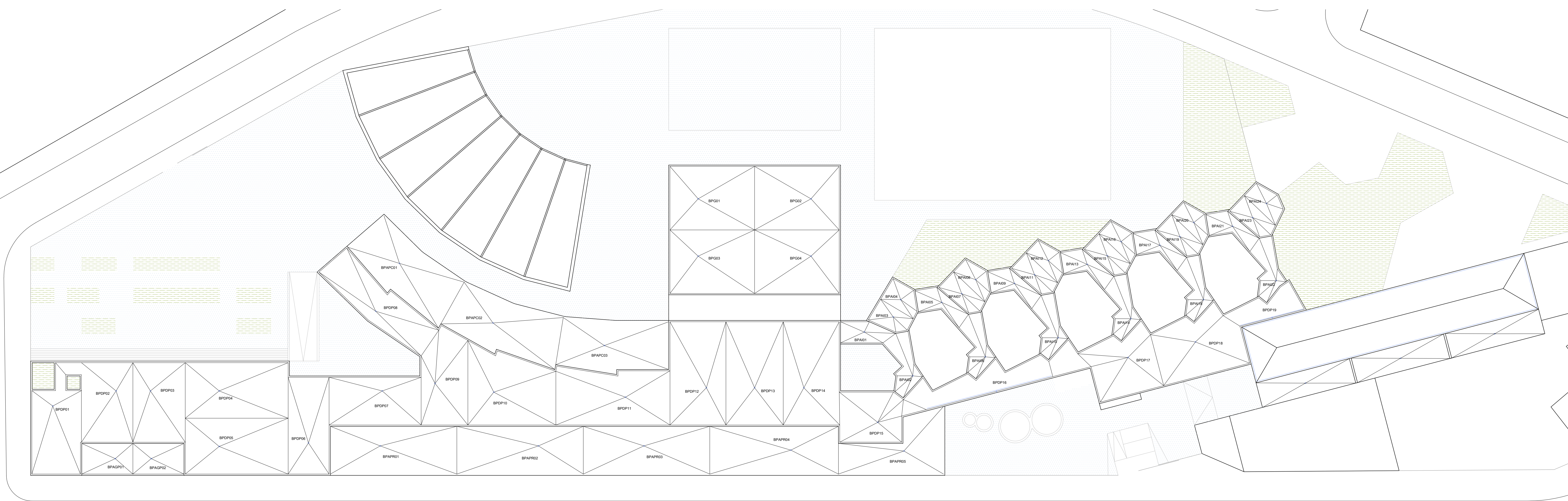
0 5 10 20 Planta baja: bajantes de aguas pluviales y residuales
