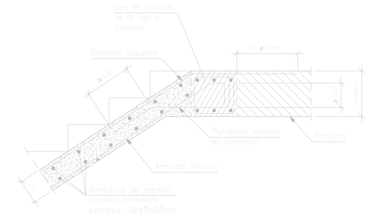
Detalle entrega zanca en viga embebida en forjado e 1,20
