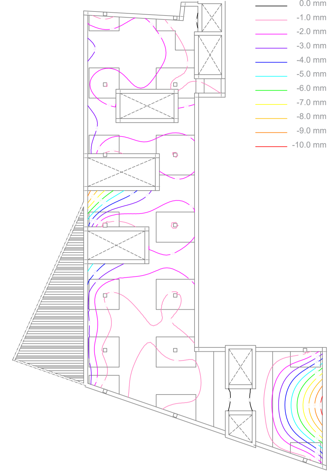
Comprobación desp. eje Z (Planta primera) CYPE 2014
