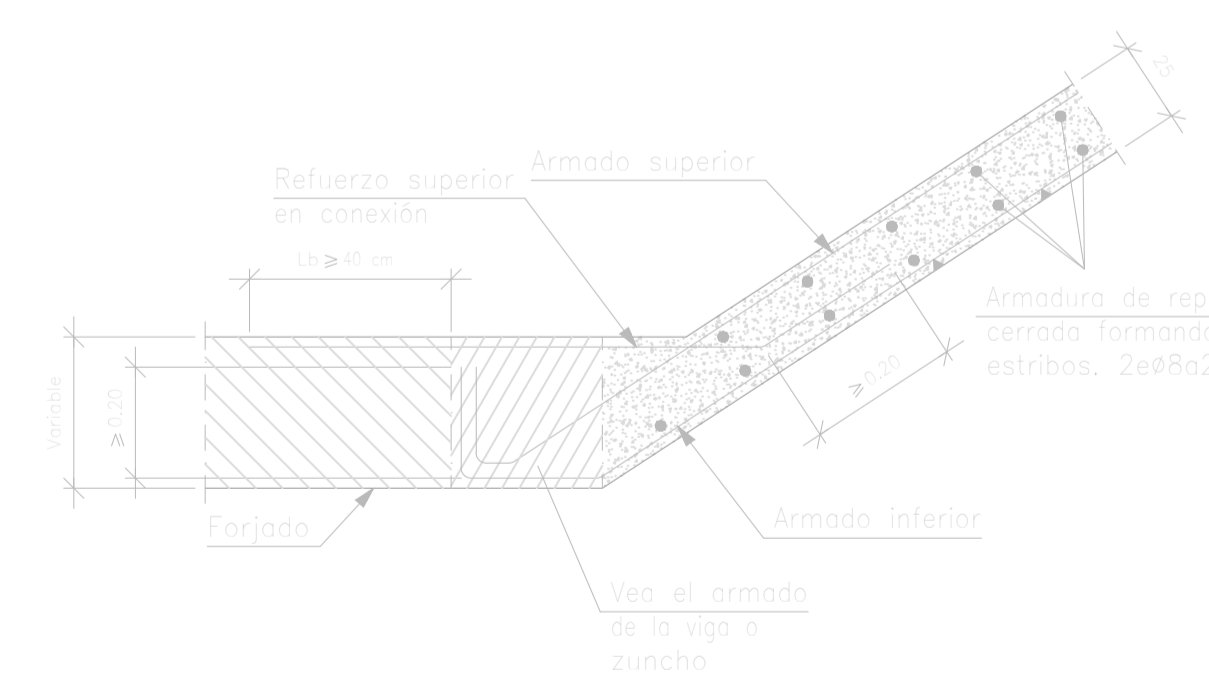
Detalle entrega zanca en viga embebida en forjado e 1,20
