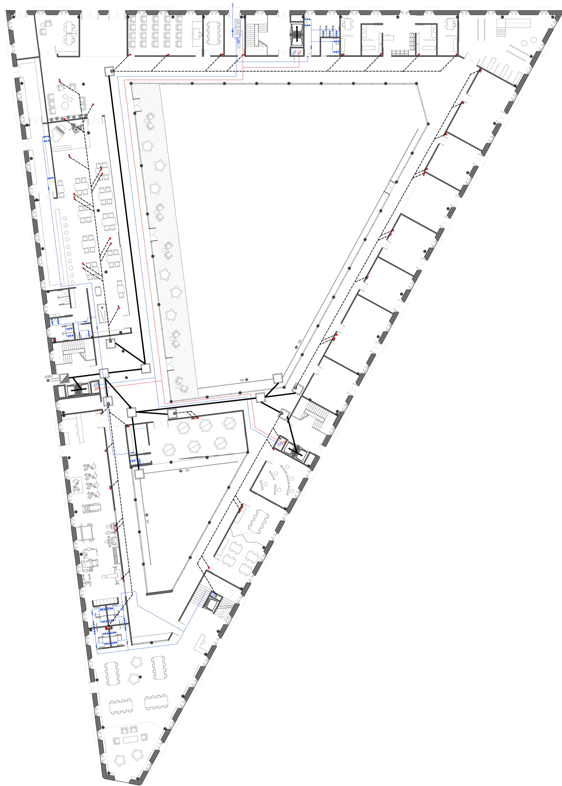
PLANTA BAJA SANEAMIENTO ESCALA 1/250
