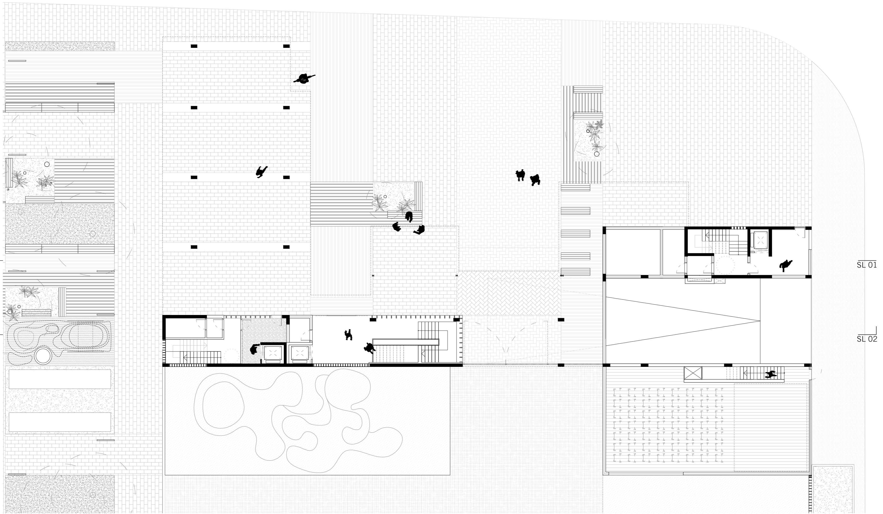
PLANTA BAJA- Accesos
