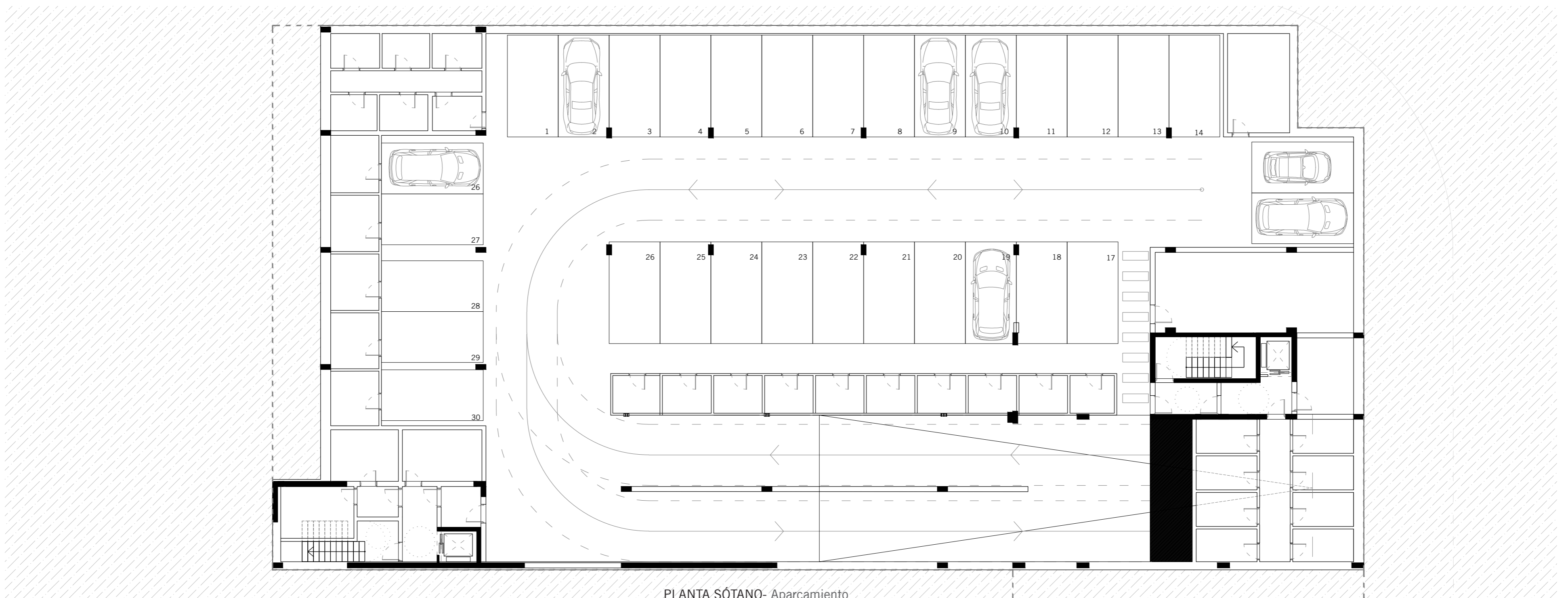
PLANTA SÓTANO- Aparcamiento
