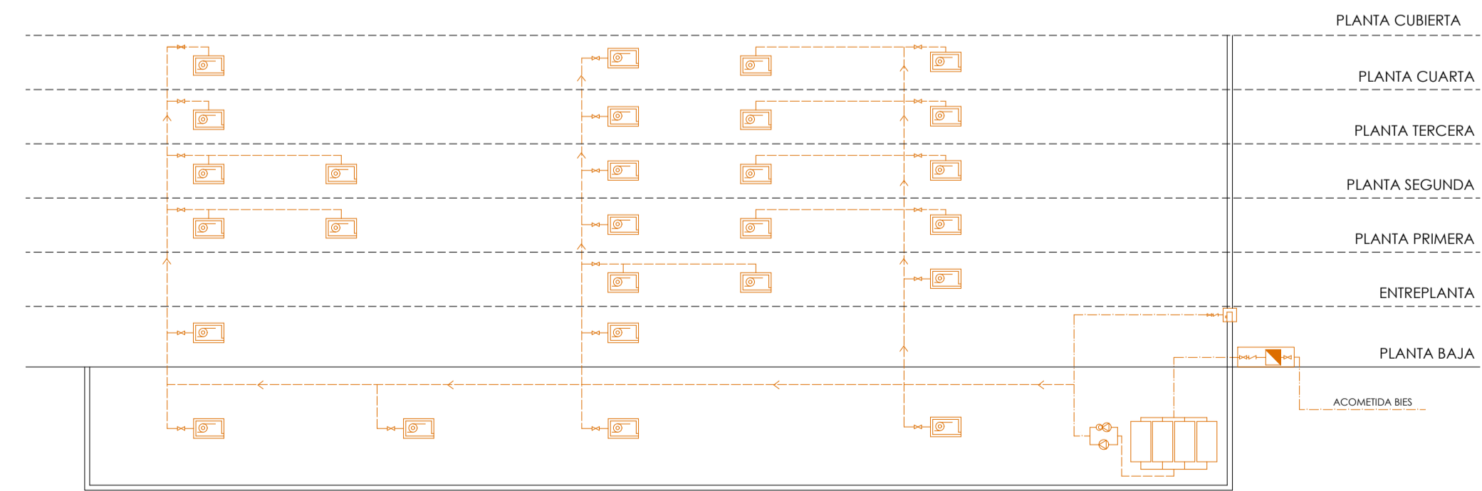
ESQUEMA DE PRINCIPIO BIES
