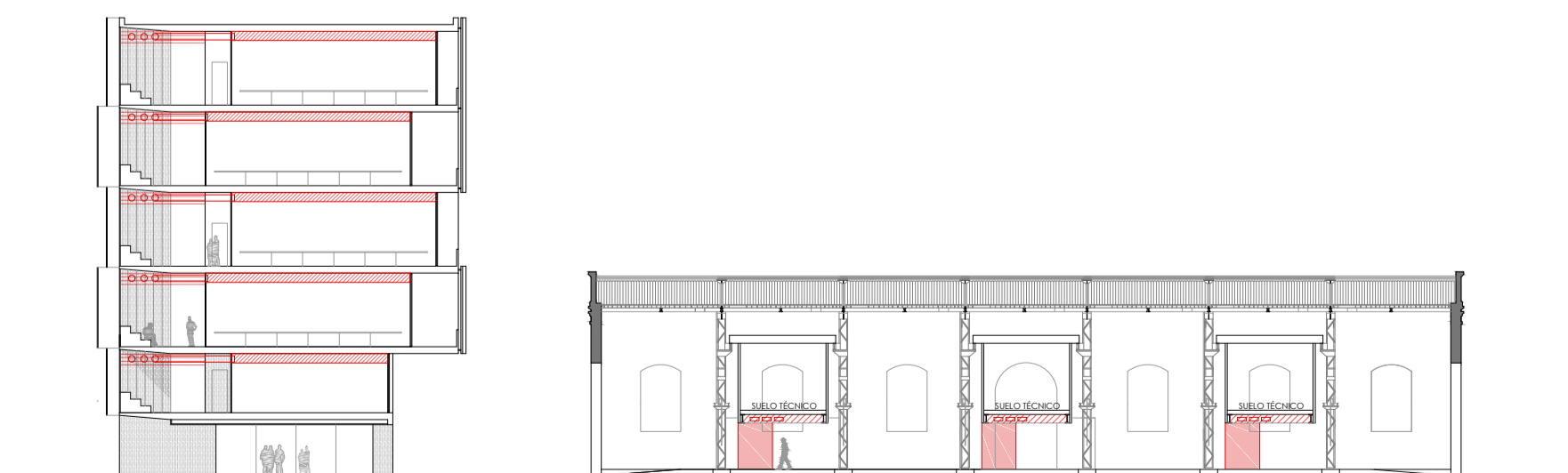
SECCIÓN TRANSVERSAL DEL EDIFICIO PRINCIPAL Y MEDIATECA DE LA NAVE CENTRAL IDENTIFICACIÓN DE CONDUCCIONES INSTALACIONES (ESCALA 1:500)
