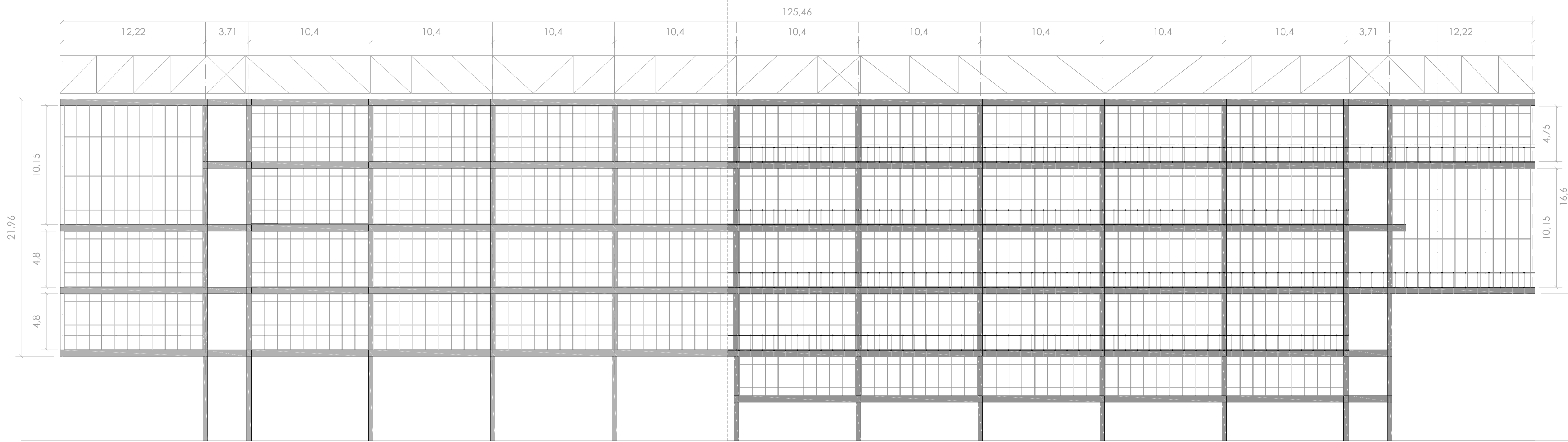
ALZADO OESTE DEL EDIFICIO PRINCIPAL_ SUBESTRUCTURA DE VIDRIO Y SUBESTRUCTURA DEL PANEL COMPOSITE
