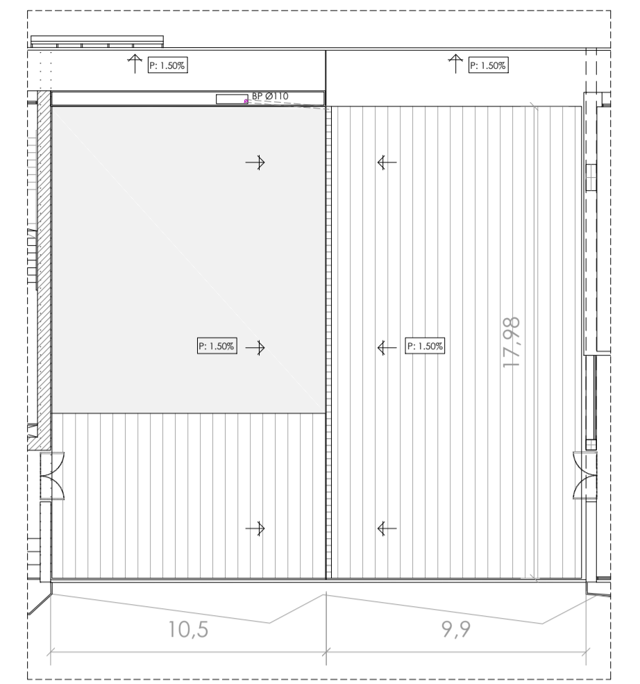
PLANTA TERCERA_ CUBIERTA DE PATIO EXTERIOR
