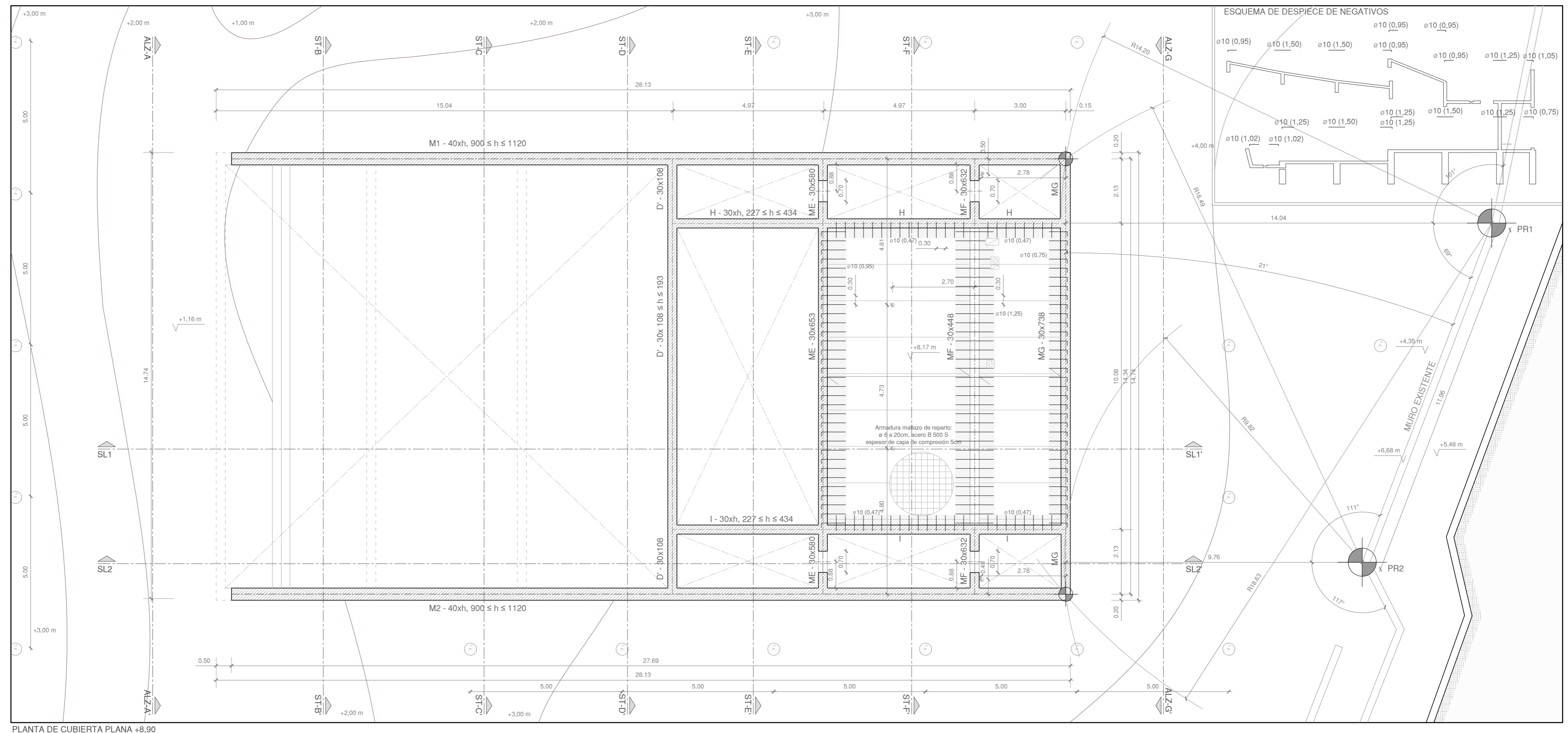
PLANTA DE CUBIERTA PLANA +8.90 Propuesta 1/100 Cotas en metros
