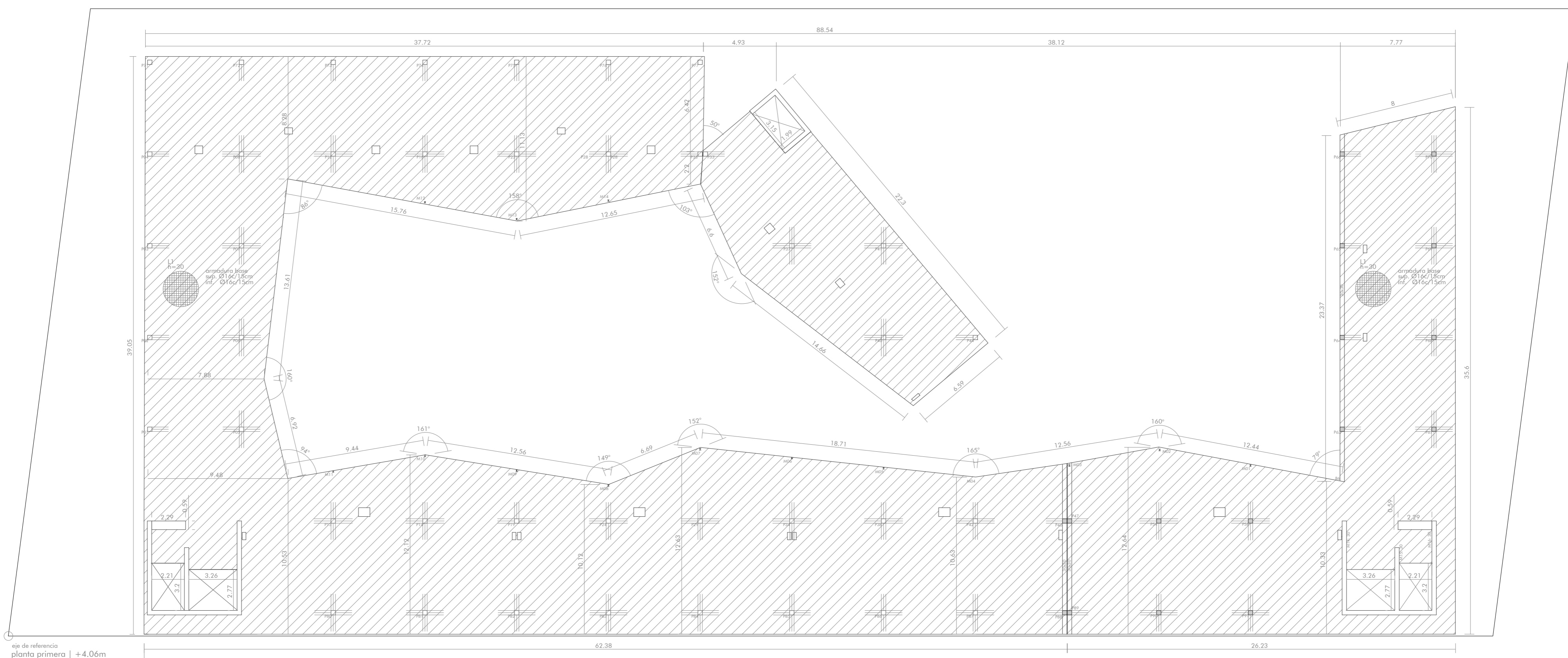
esp. de referencia planta primera | +4.06m
