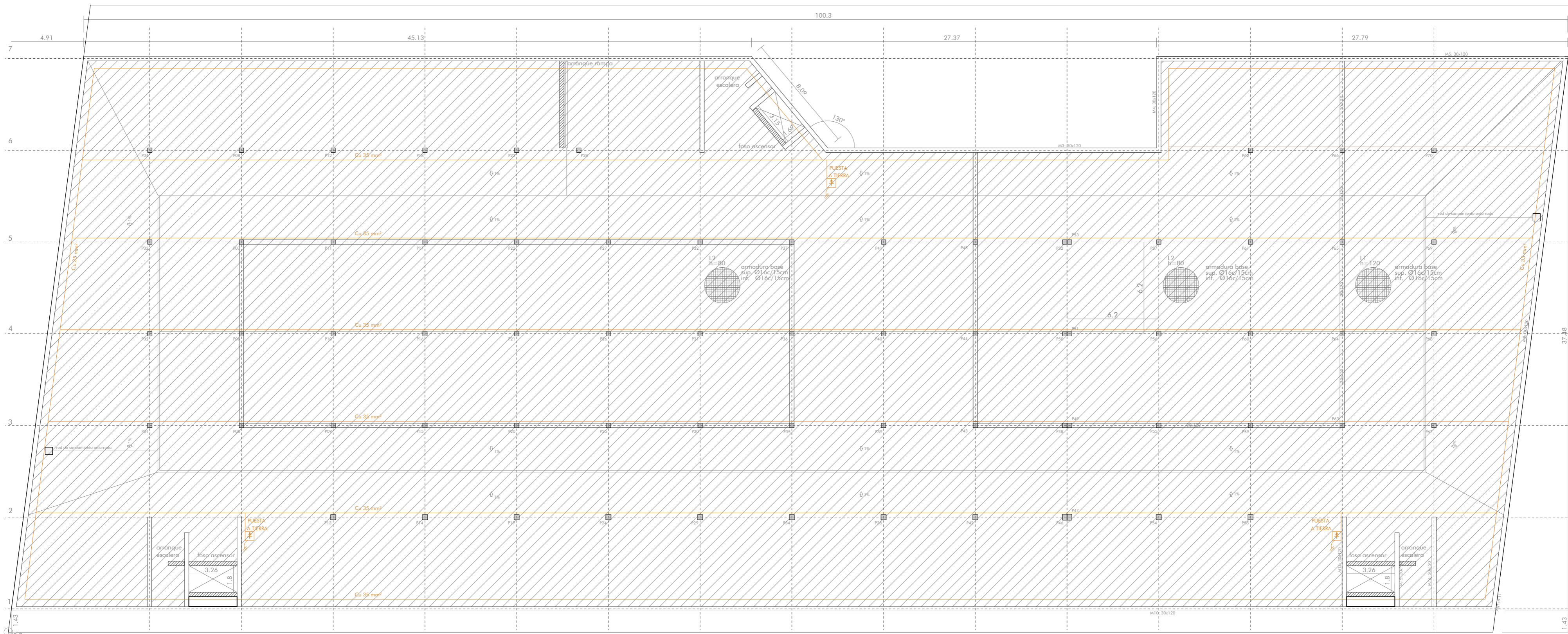
esp. de referencia planta cimentación | -3.75m
