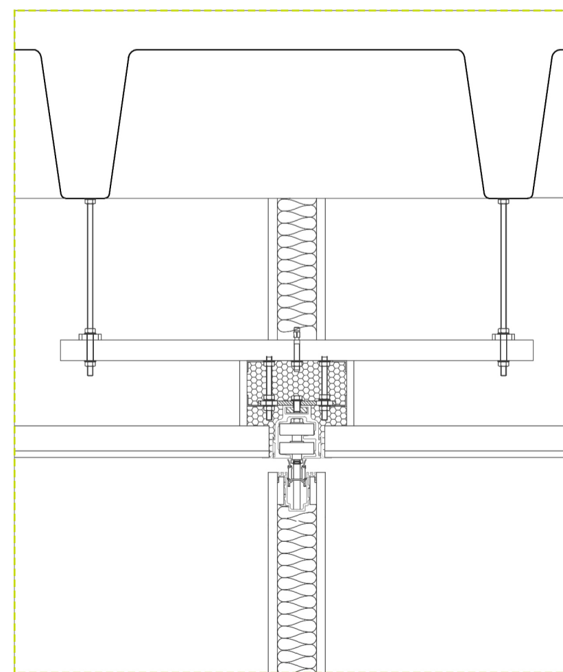
CUBIERTA NO TRANSITABLE E:1/10
