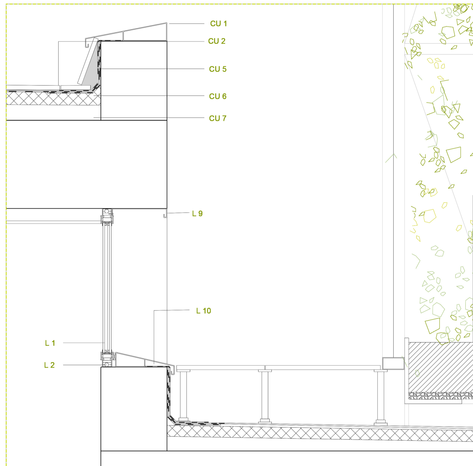
CUBIERTA NO TRANSITABLE E:1/10
