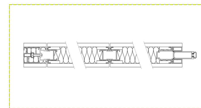
PANEL ACÚSTICO MOVIL E:1/10
