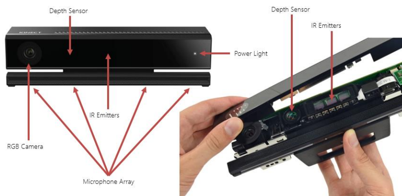
Figura 2-1. Localización de los distintos sensores en la Kinect v2 (9)
