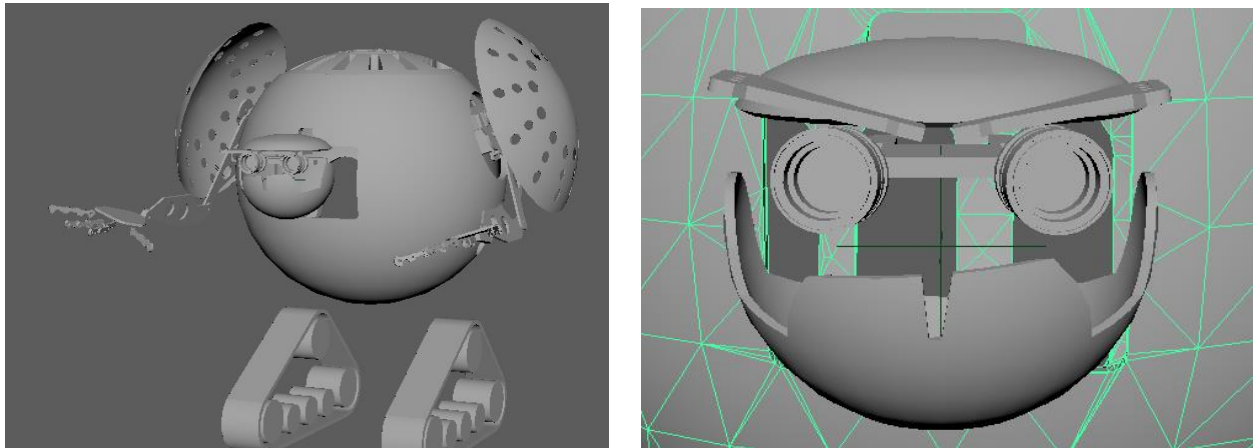
a) Visualizado del cuerpo entero del robot
