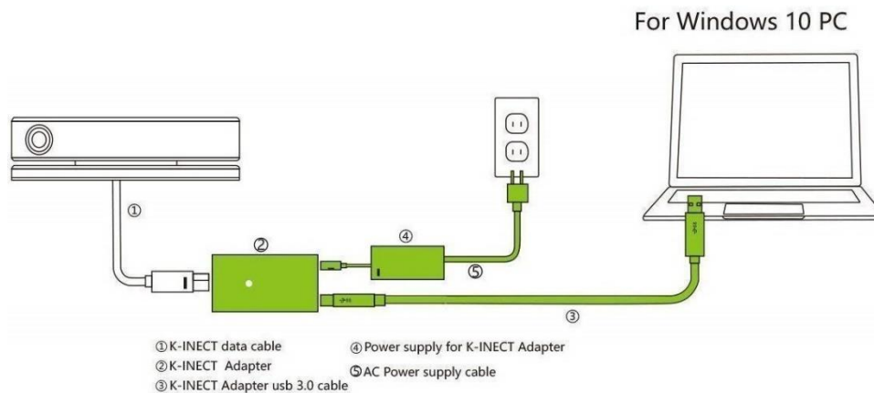
Figura 2-2. Esquema de cables y hubs del adaptador de Kinect v2 para Windows (13)
