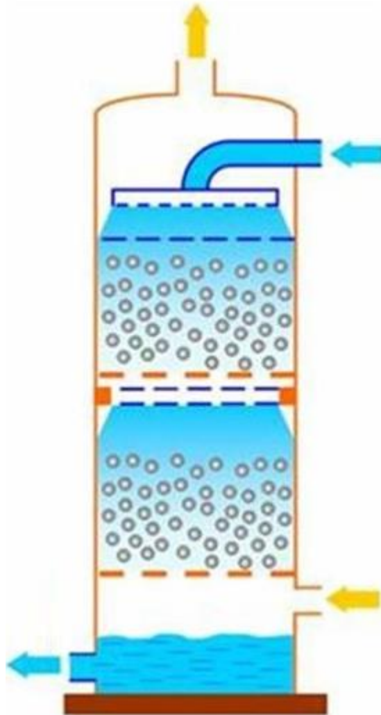
Figura 4-23. Esquema de una torre de lavado (Ingenieromarinero.com, 2019)
