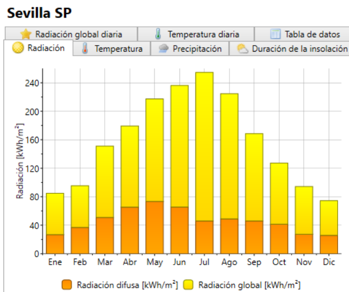
Ilustración 16: Gráfico obtenido por Meteonorm 7.3 de la radiación solar en Sevilla
