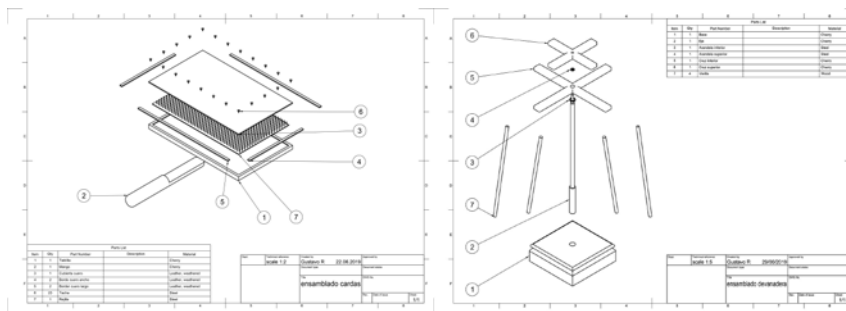
Fig. 8. Plano ensamblado: Herramienta carda y devanadera, 2019. Gustavo Hilario Rebozo Morales.
